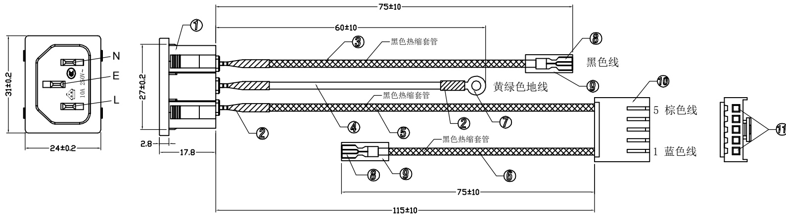
焊接(钩焊)示意图
