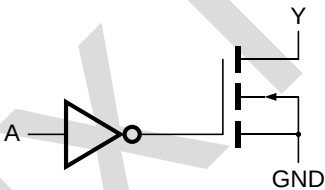
图2 逻辑框图
