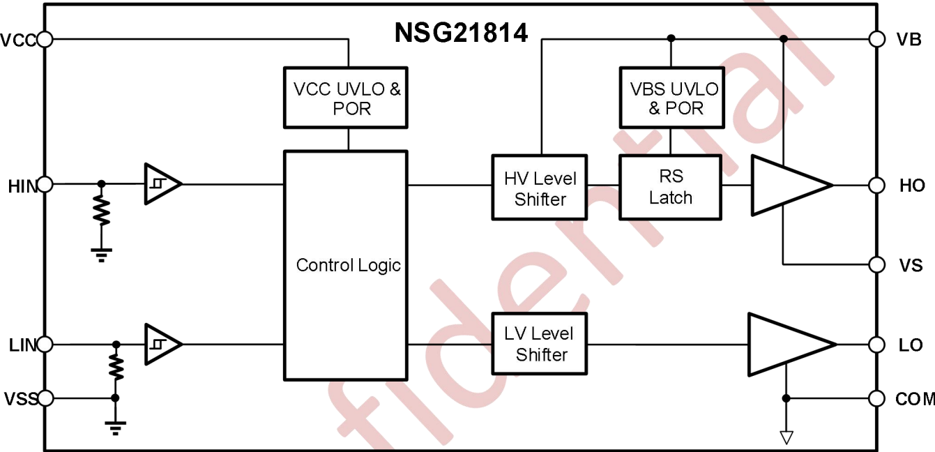
图 10-1 NSG21814 功能框图
