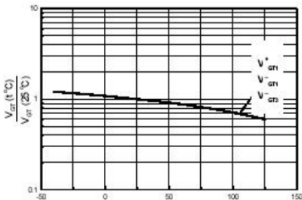
结温 (°C)
