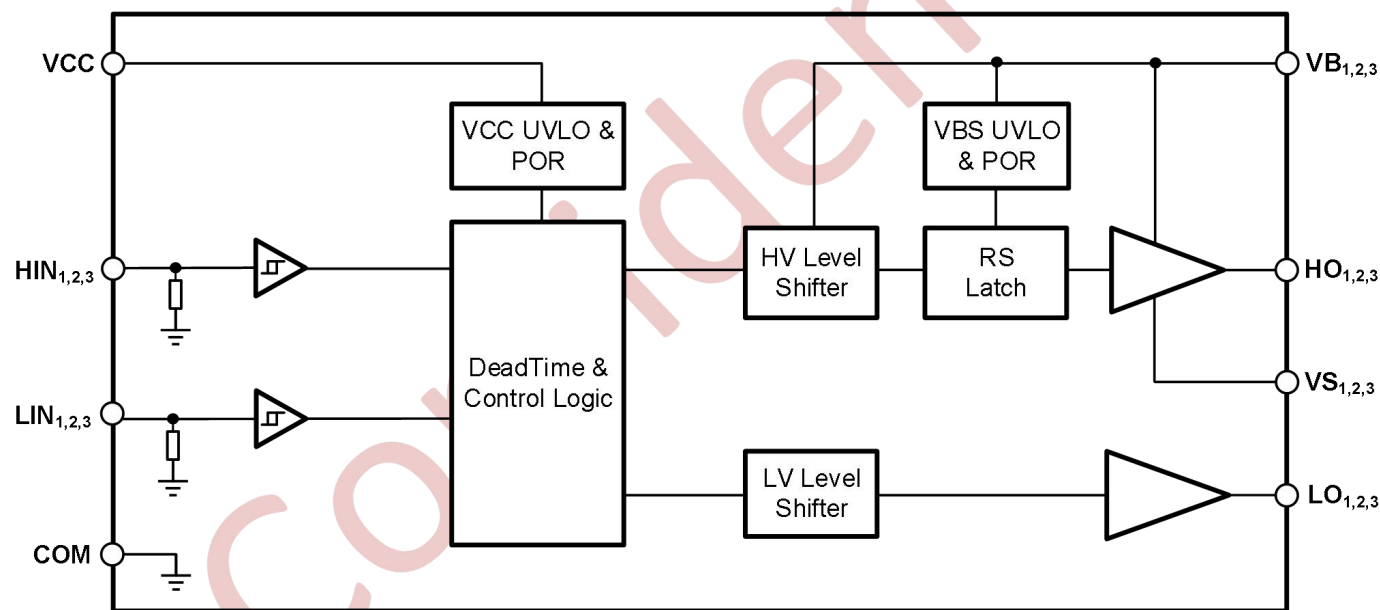
图 10-1 G2061 功能框图
