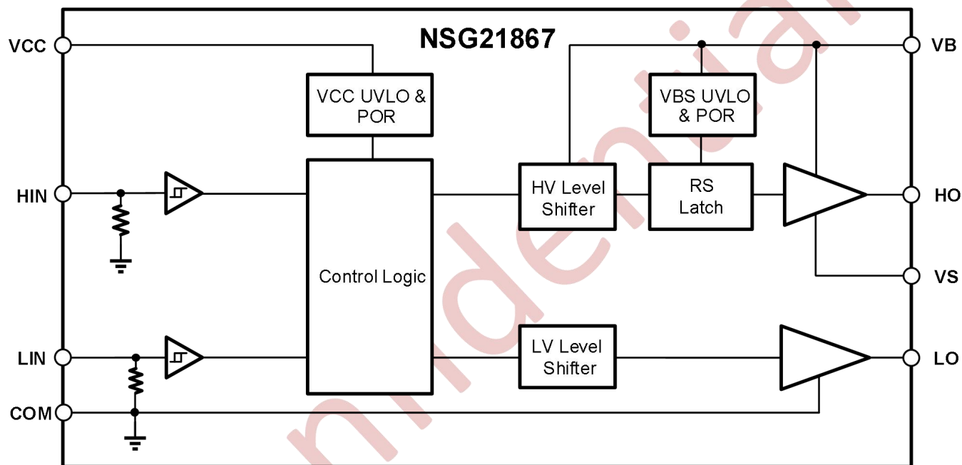
图 10-4 NSG21867 功能框图
