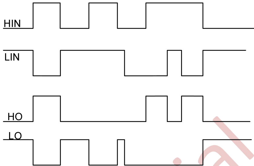
图 9-1 NSG2024 输入输出时序波形
