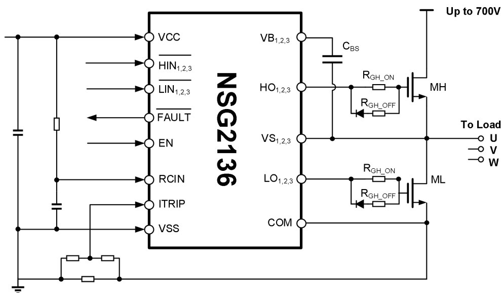
图 10-7 典型应用电路图
