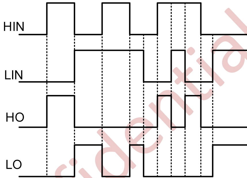
图 9-1 输入输出时序波形
