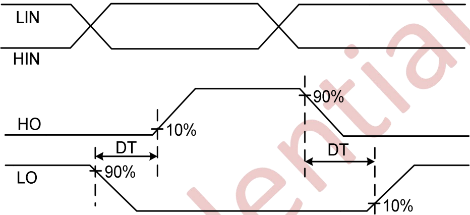
图 9-3 死区时间波形定义
