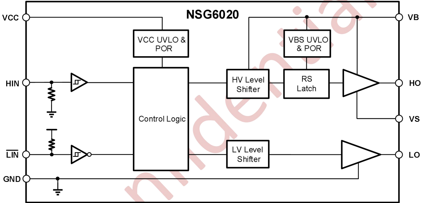
图 10-4 NSG6020 功能框图
