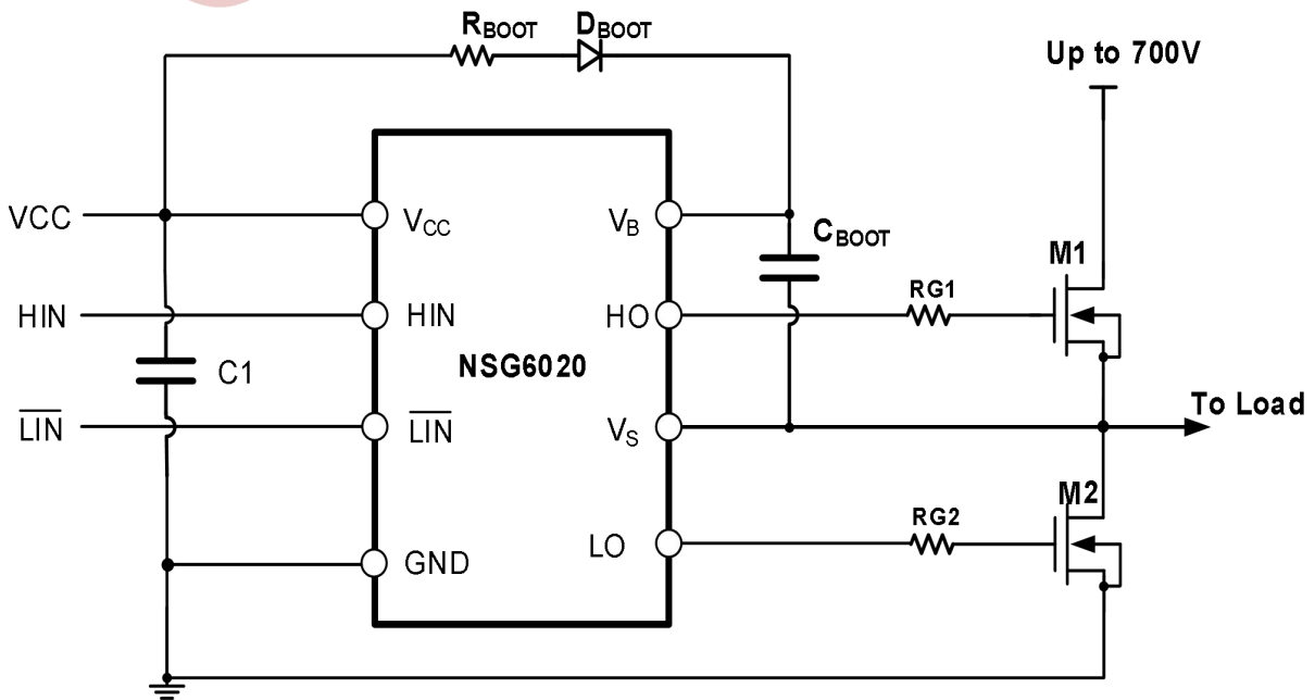
图 10-2 典型应用电路图
