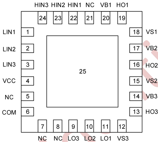
图 7-1 NSG2065Q QFN24 顶视图
