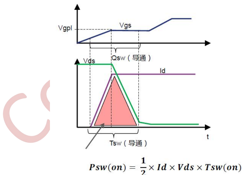
图 11-3 阻性负载条件下的 MOS 开关损耗
