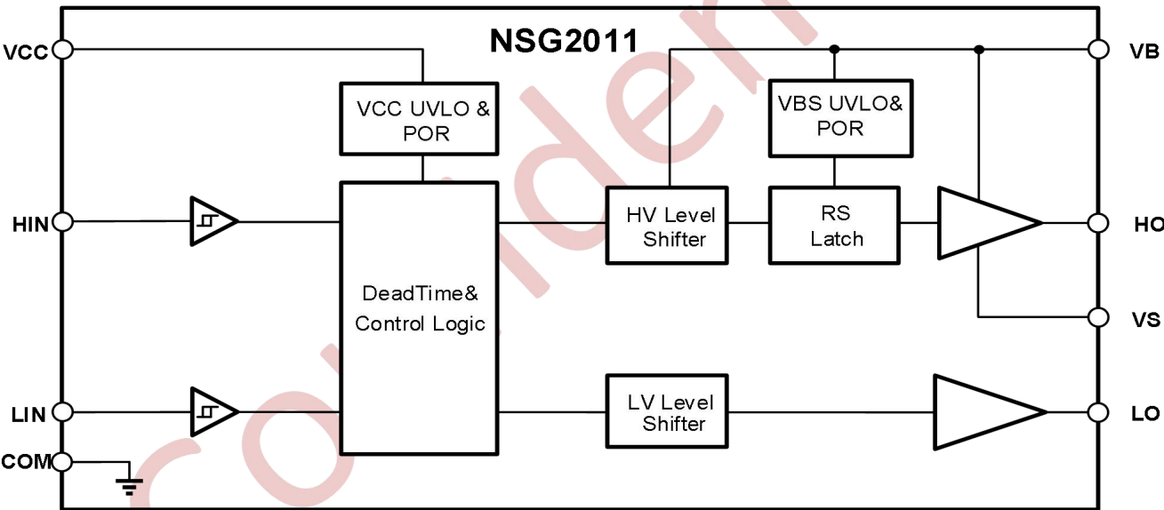
图 10-1 NSG2011 功能框图
