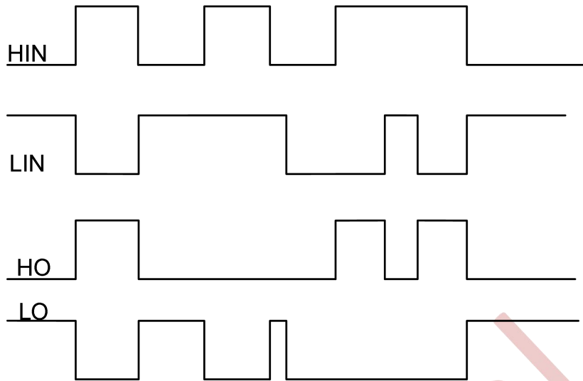
图 9-1 NSG2011 输入输出时序波形
