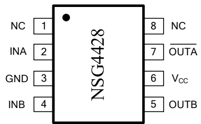
图 7-1 8-脚 SOIC8 顶视图
