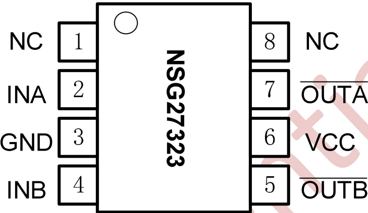
图 7-1 8-脚 SOP8 顶视图
