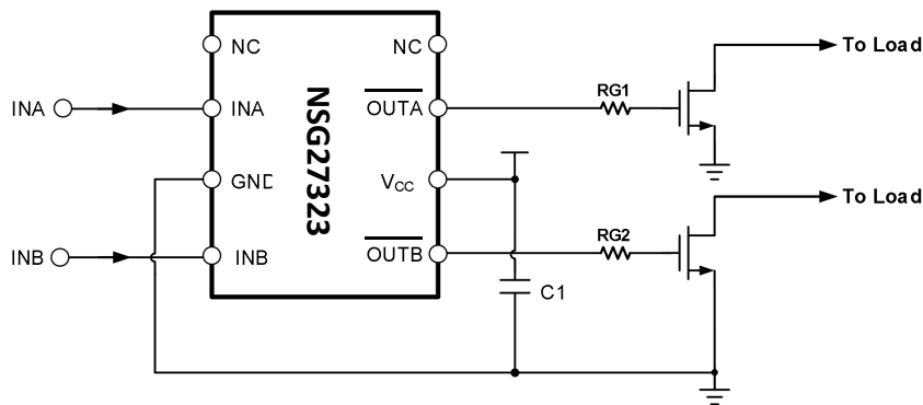
图 10-2 NSG27323 反相典型应用电路图
