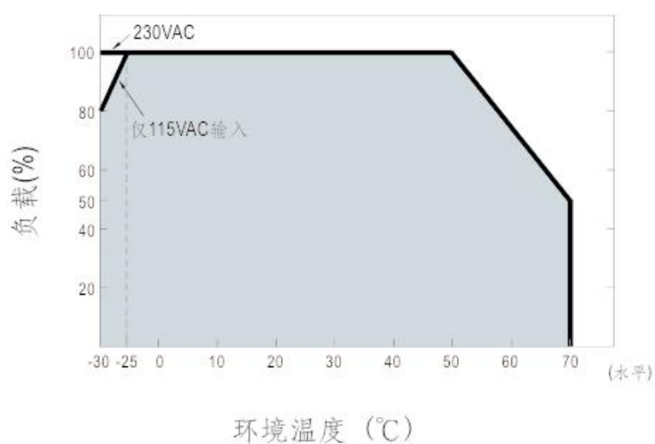
■ 减额曲线
