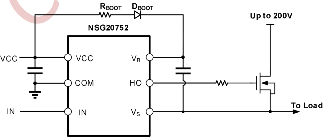
图 10-2 典型应用电路图
