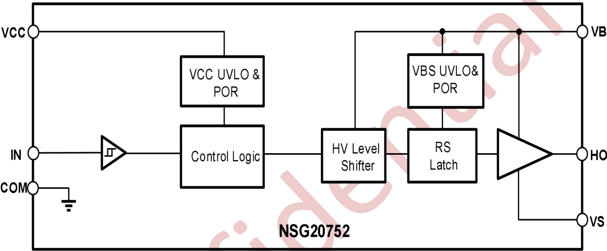
图 10-1 NSG20752 功能框图
