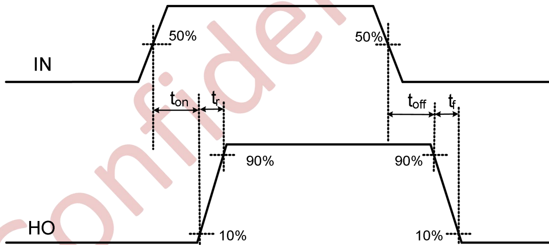
图 9-2 开关波形定义
