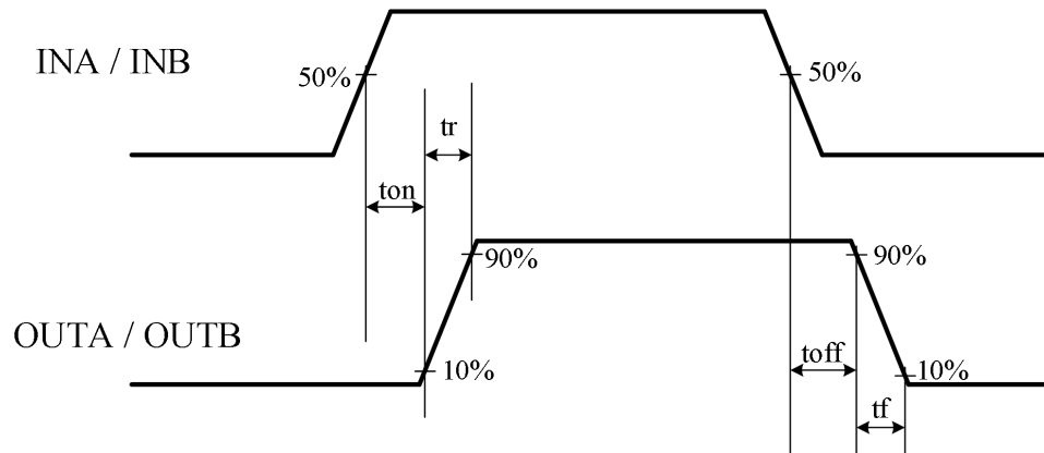
图 9-1 输入输出延时波形图
