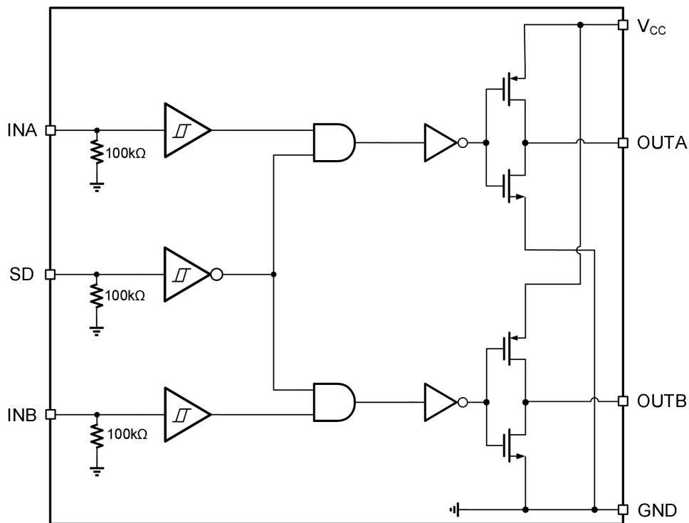
图 10-1 NSG4437 功能框图
