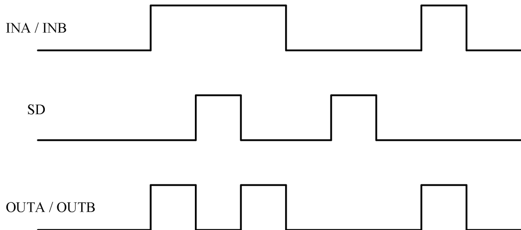
图 9-2 输入输出逻辑功能图
