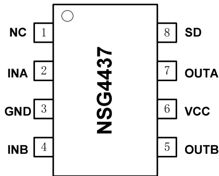
图 7-1 8-脚 SOP8 顶视图
