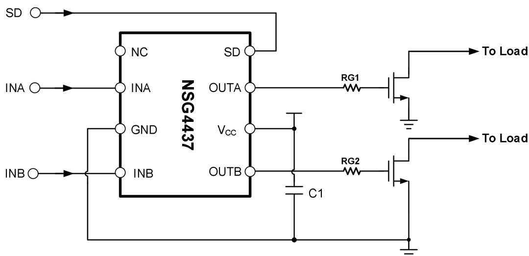
图 10-1 NSG4437 典型应用电路图
