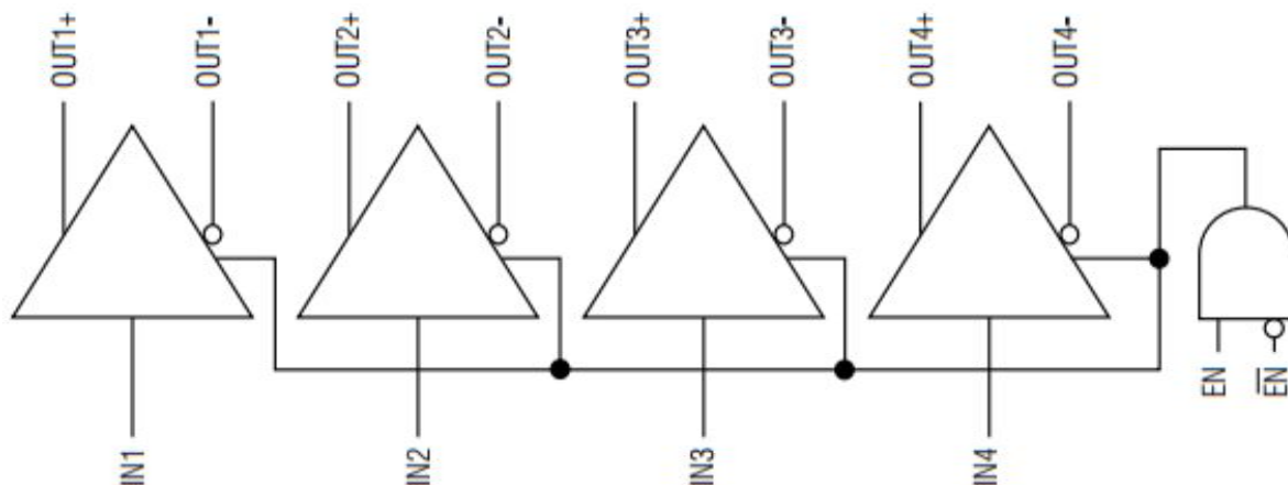
图3 功能框图
