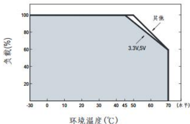
■ 减额曲线
