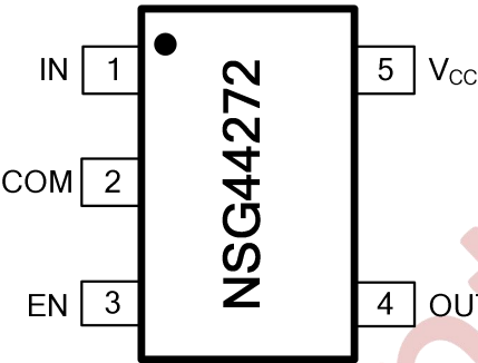
图 6-1 5 脚 SOT23-5 顶视图
