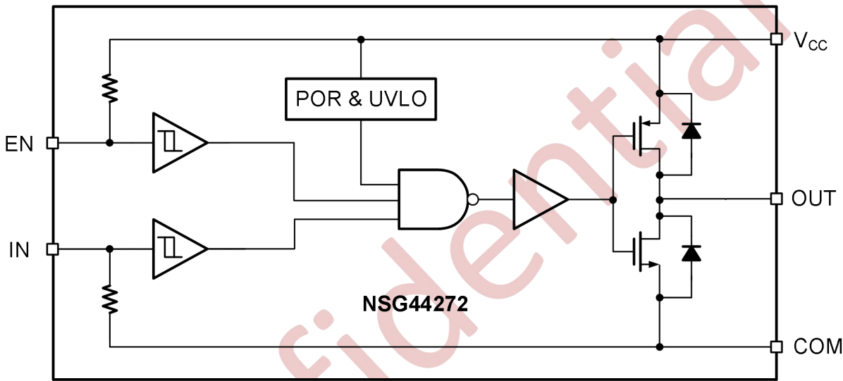
图 9-1 NSG44272 功能框图
