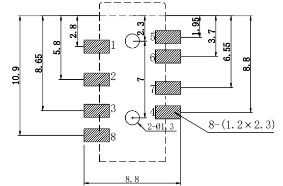
线路板开孔尺寸
