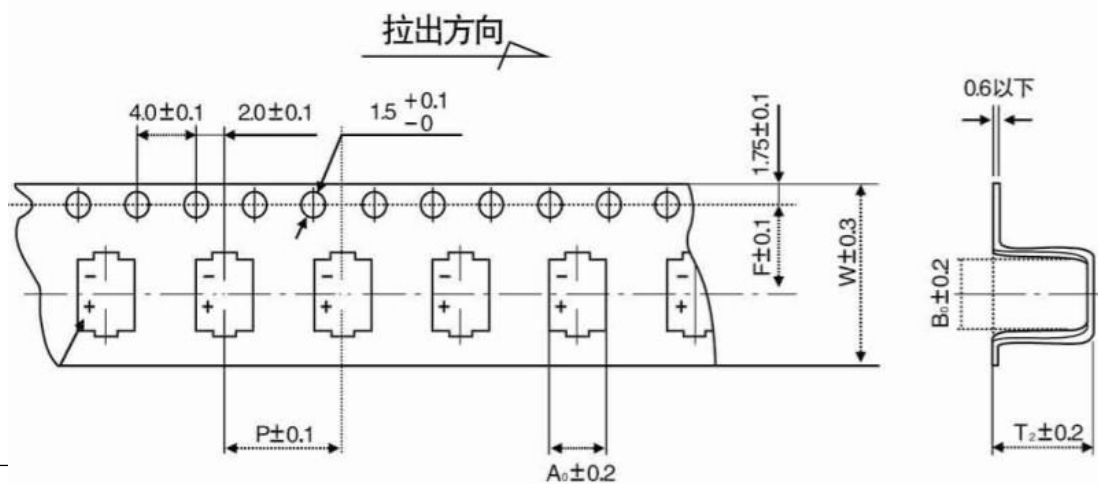
Fig.1 (Ø4 ~ Ø10)
