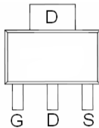
SOT223
