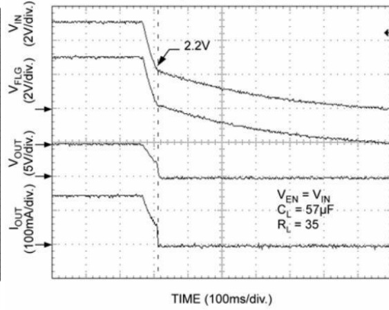
UVLO- V_{IN} Falling (XL2026-1)
