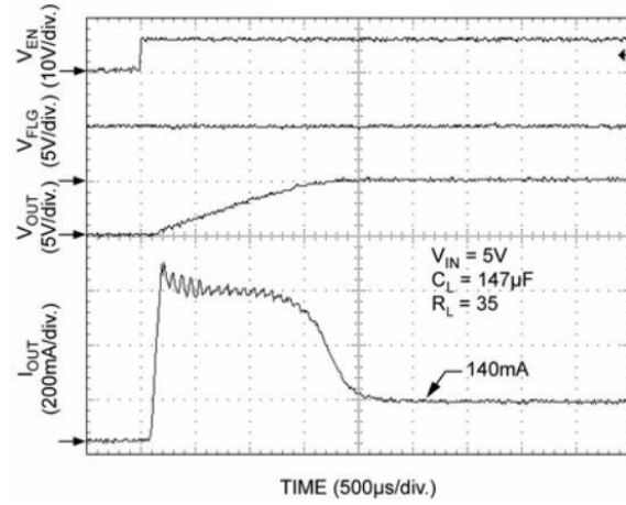
Turn-On (XL2026-1)
