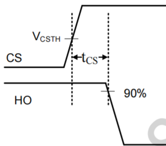
图 6-4 CS 关断时间定义
