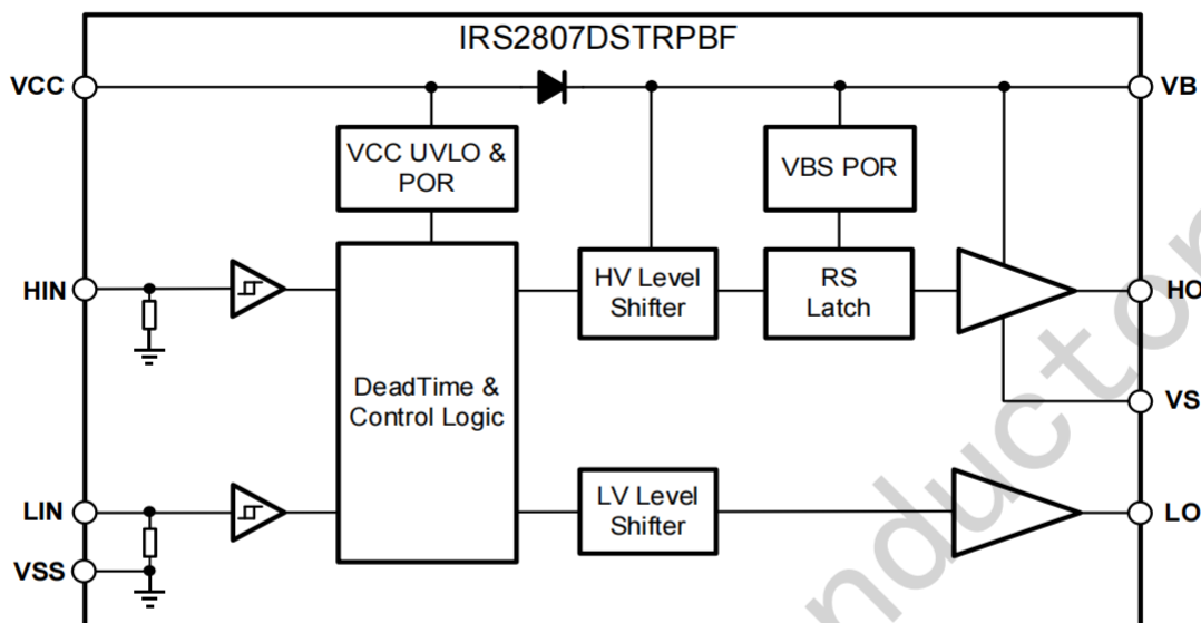
图7-1 IRS2807DS的功能框图
