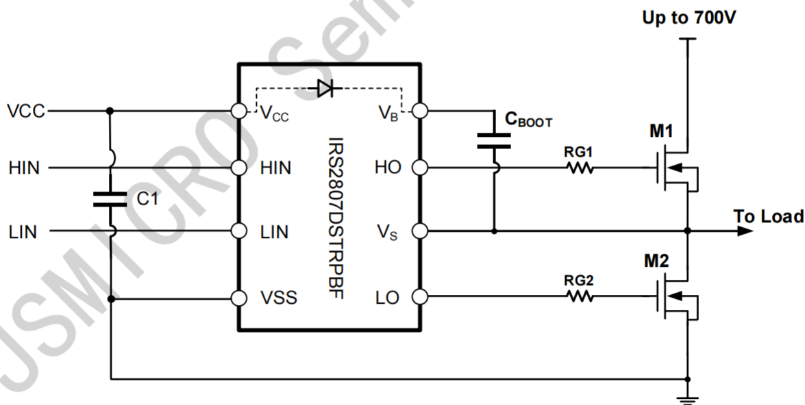
图7-2 IRS2807DS典型应用电路图
