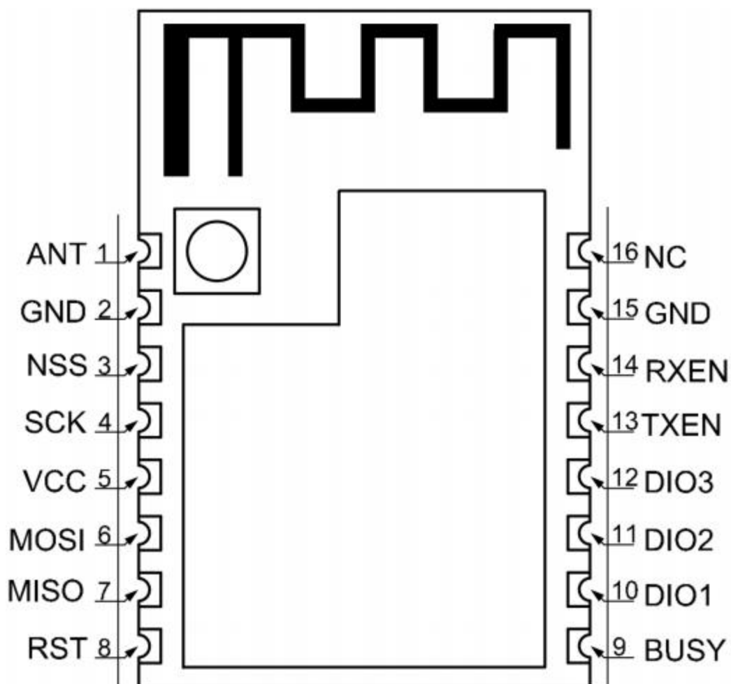
图 1-1 俯视图
