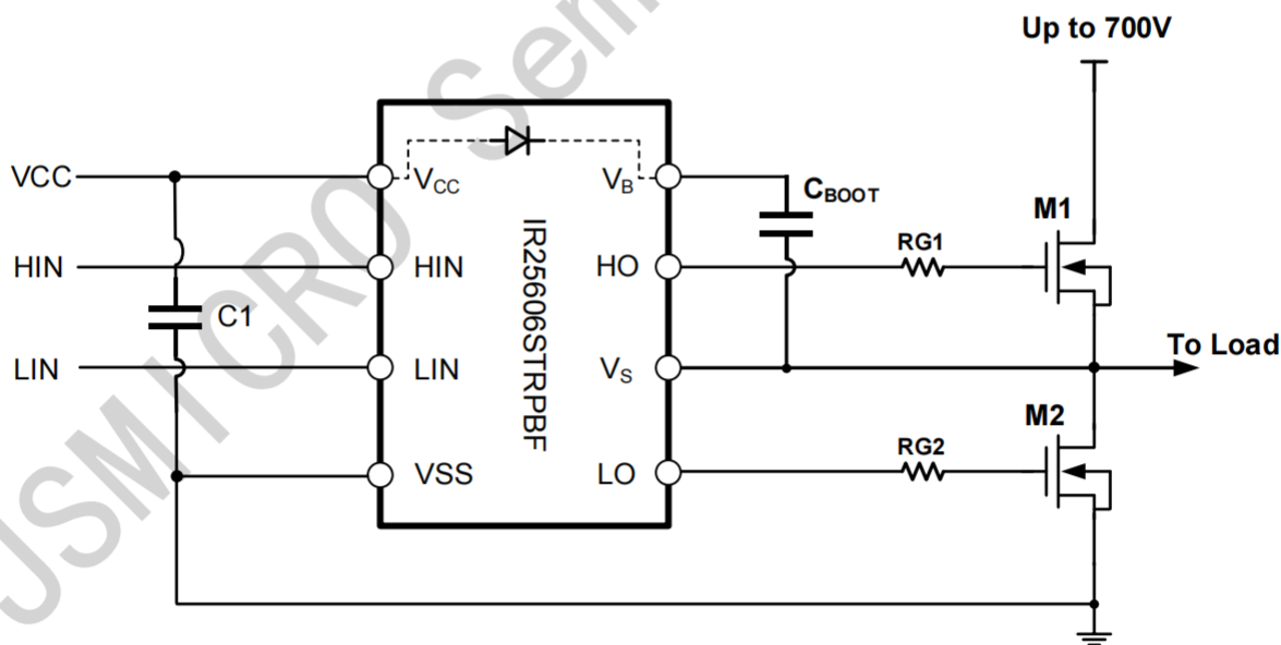
图7-2 IR25606S典型应用电路图
