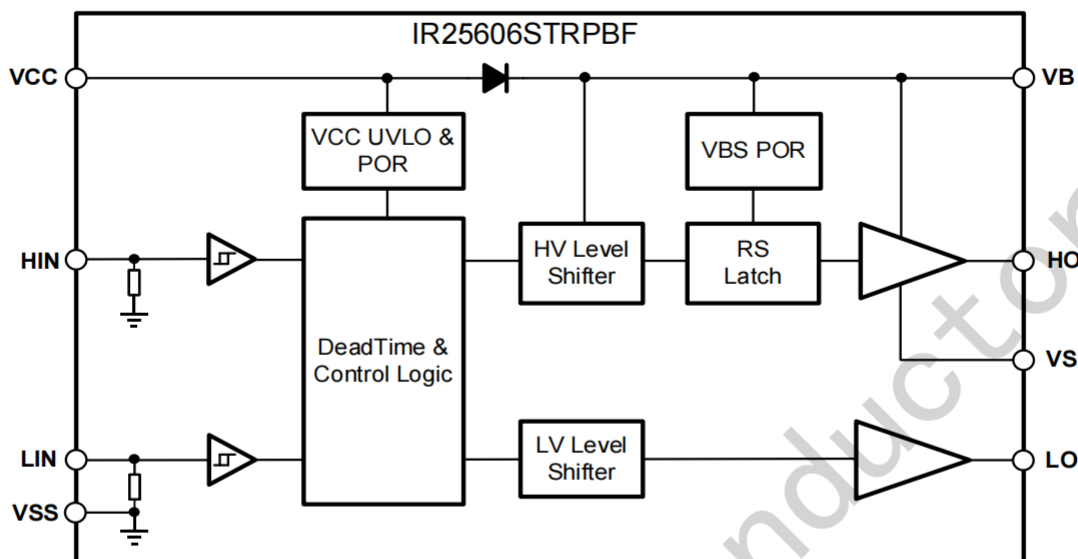
图7-1 IR25606S的功能框图
