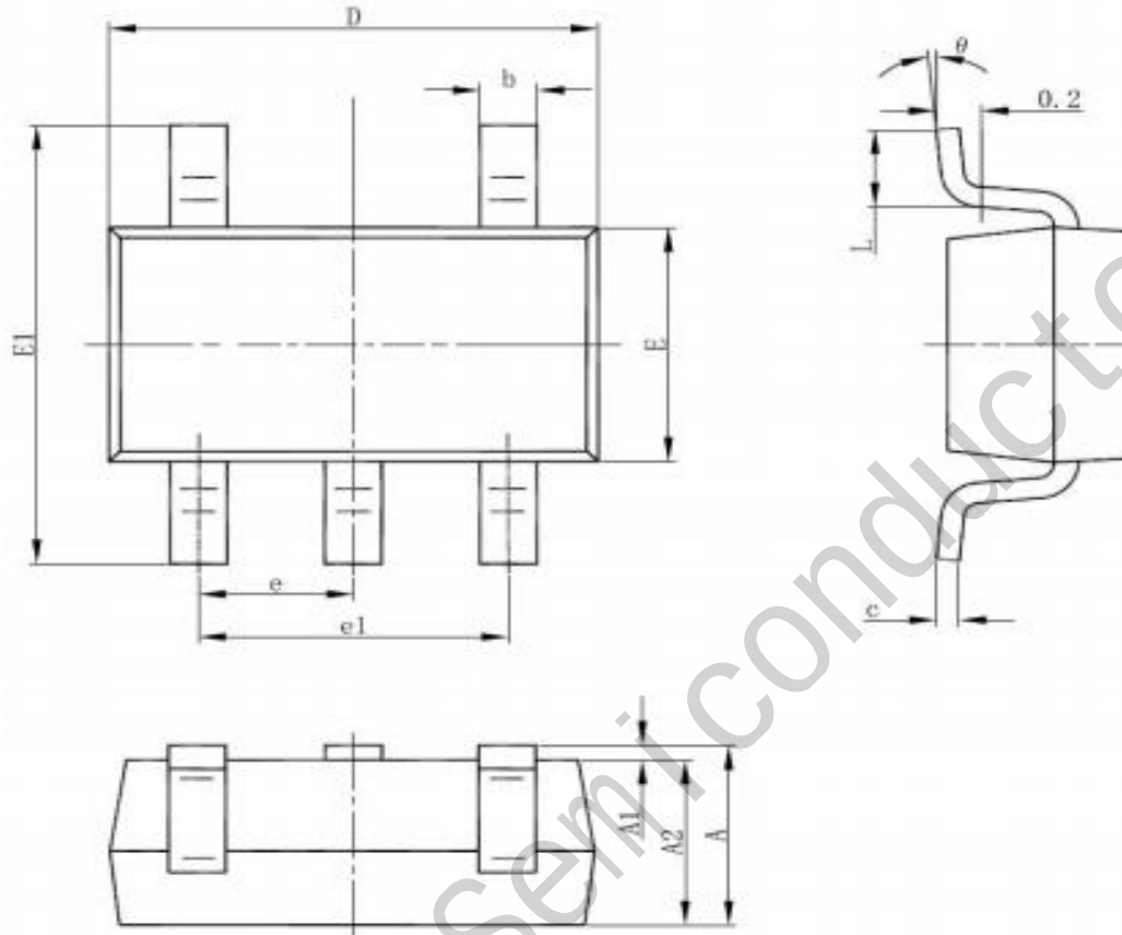
SOT23-5 封装外形尺寸
