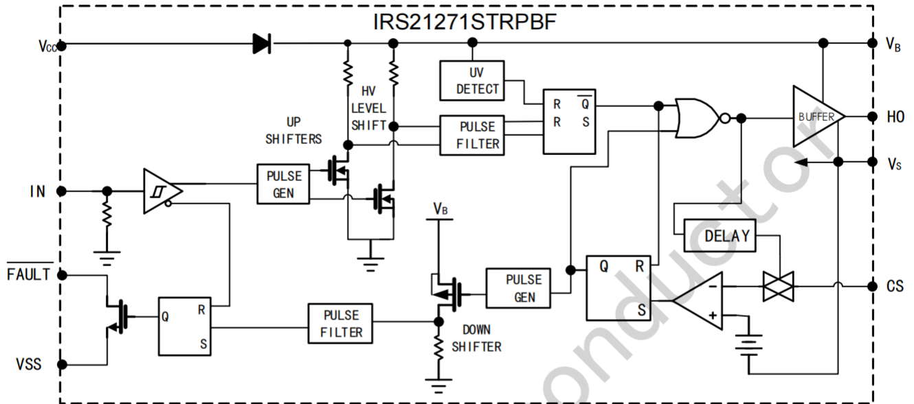
图 7-1 功能框图
