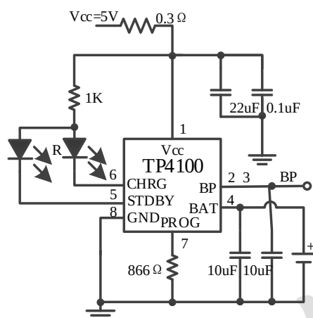
TP4100 带耗散电阻
