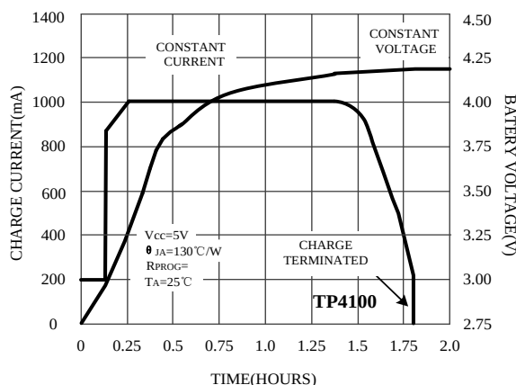
1A 电流完整的充电循环 (1000mAh)
