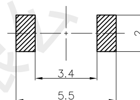
安裝參考尺寸
