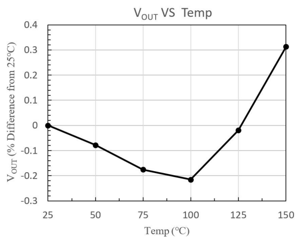
图 4 输出电压随温度变化( V_{IN}=10V , I_{OUT}=10mA )
