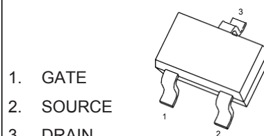
SOT-323
