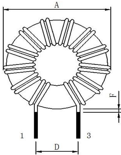
1. 正视图
