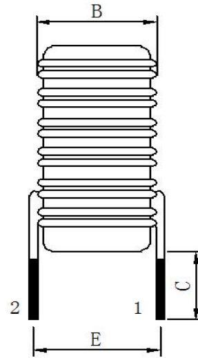
2. 侧视图
