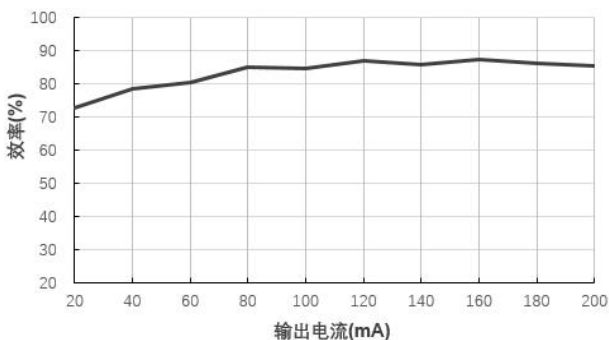
效率 VS 输出电流 B2405XT-1WR3@Vin=24V
