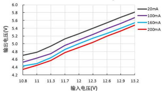
输出电压 VS 输入电压 B1205XT-1WR3@Vin=12V
