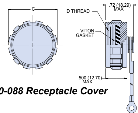
660-087 & -088 Dimensions
