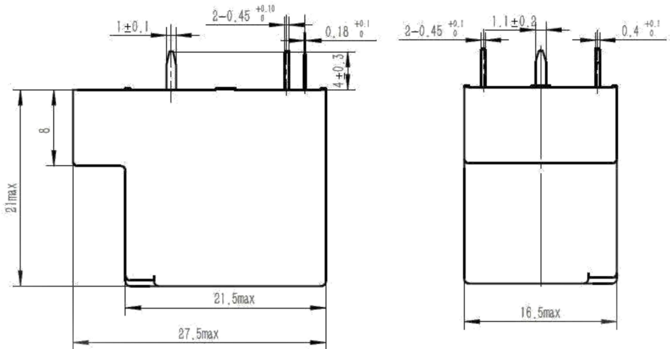
外形图
