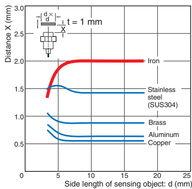
E2E-X10D□/-X10T1
