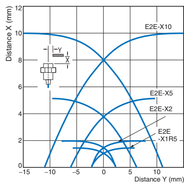
E2E-X□E□/-X□Y□/-X□F□
