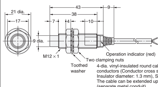
Diagram 8 E2E-X5MY□
