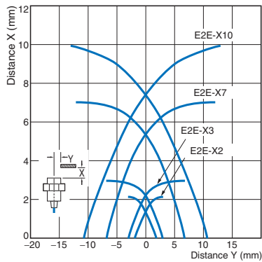
E2E-X□D□/-X□T1
