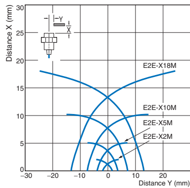
E2E-X□ME□/-X□MY□/-X□MF□
