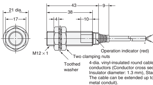
Diagram 7 E2E-X2Y□
