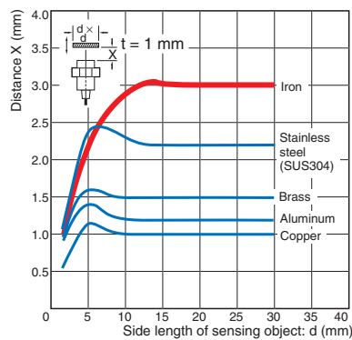
E2E-X4MD□
