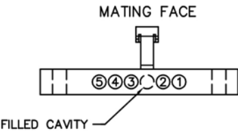
RECEPTACLE MA-121-005-261-A03WA
