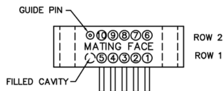
RECEPTACLE MA-261-010-435-A6300
