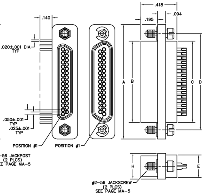
RECEPTACLE
