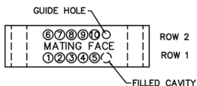
PLUG MA-211-010-161-A66WA
