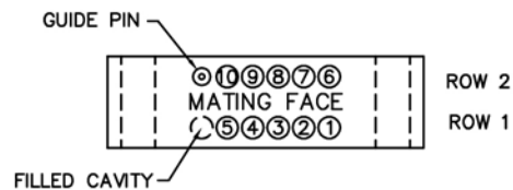
RECEPTACLE MA-221-010-261-A63WA
