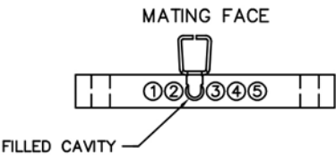
PLUG MA-111-005-161-A03WA
