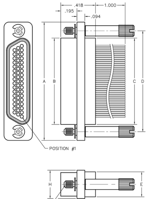
RECEPTACLE
