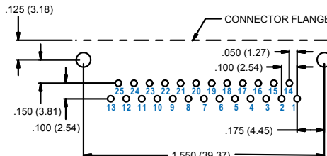
25 PIN M83513/16-D
