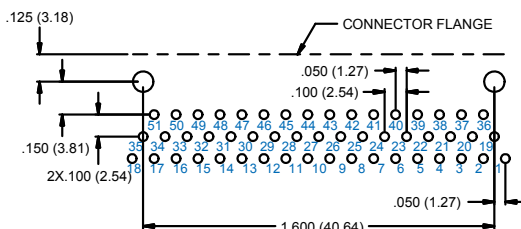
51 PIN M83513/17-G
