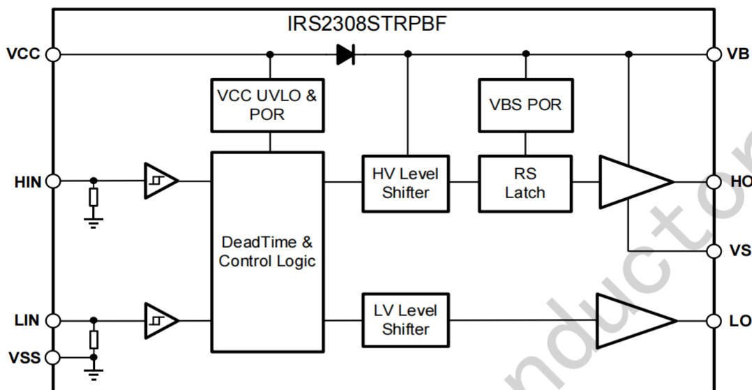
图7-1 IRS2308S的功能框图
