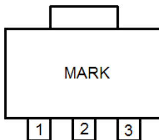
SOT-89
