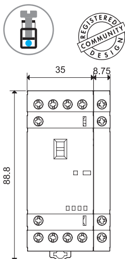
Type 22.34 + 022.33/022.35 Box clamp
