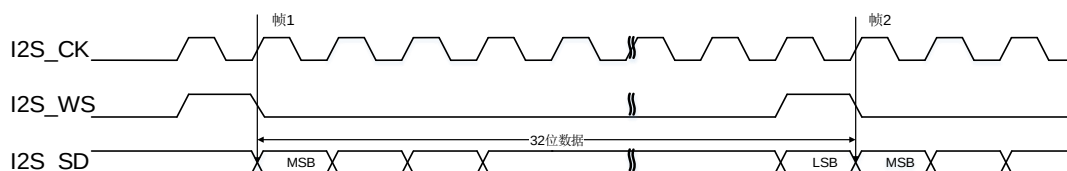
图 22-39. PCM 标准短帧同步模式时序图 (DTLEN=10, CHLEN=1, CKPL=0)
