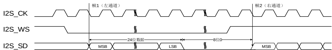
图 22-21. I2S 飞利浦标准时序图 (DTLEN=01, CHLEN=1, CKPL=0)
