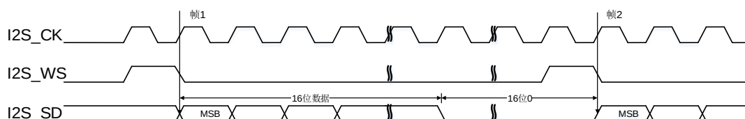
图 22-43. PCM 标准短帧同步模式时序图 (DTLEN=00, CHLEN=1, CKPL=0)
