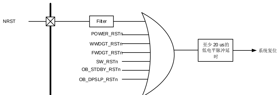
图 4-1. 系统复位电路
