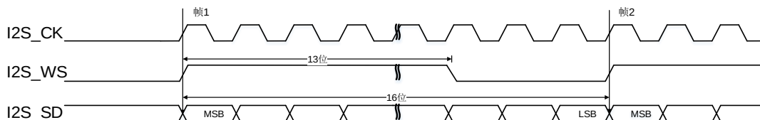
图 22-45. PCM 标准长帧同步模式时序图 (DTLEN=00, CHLEN=0, CKPL=0)
