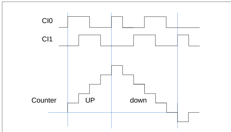
图 17-14. 编码器接口模式下计数器运行例子
