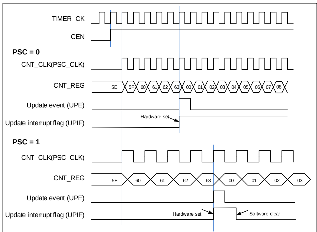
图 17-42. 向上计数时序图, PSC=0/1
