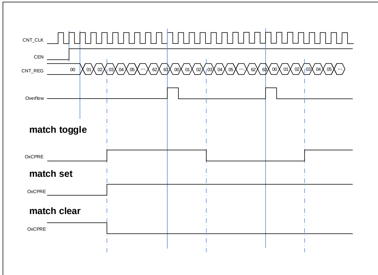
图 17-32. 三种输出比较模式
