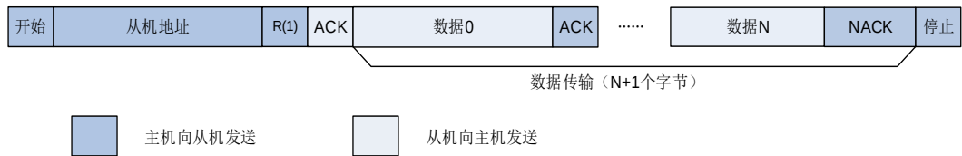
图 21-6. 7 位地址的 I2C 通讯流程（主机接收）
