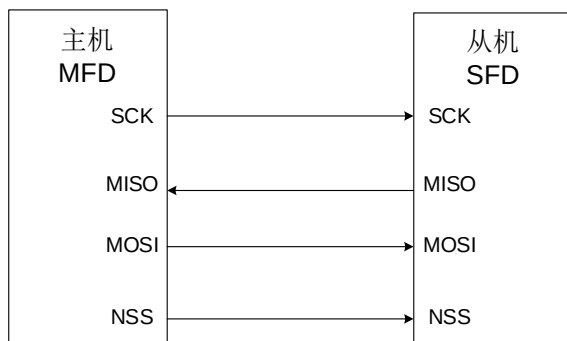
图 22-6. 典型的全双工模式连接
