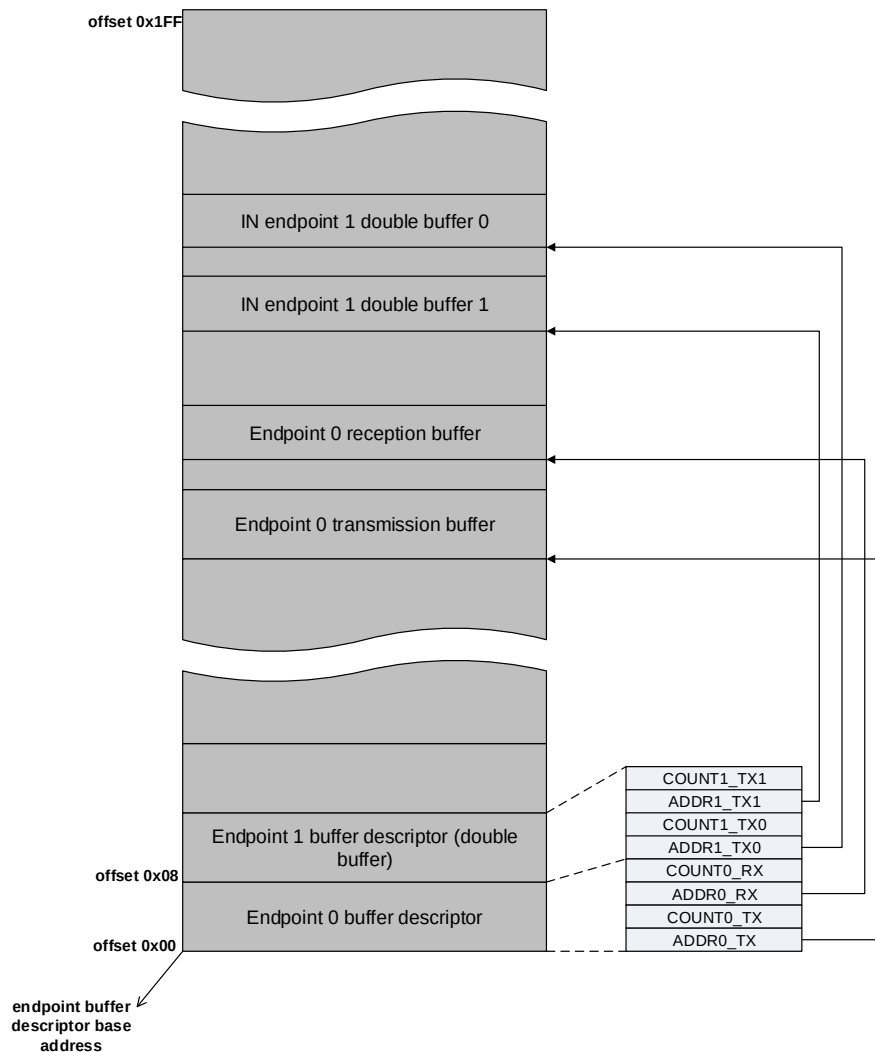
图 27-2. 缓冲描述符表的用法示例 (USBD_BADDR = 0)
