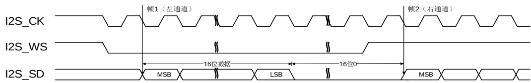
图 22-24. I2S 飞利浦标准时序图 (DTLEN=00, CHLEN=1, CKPL=1)
