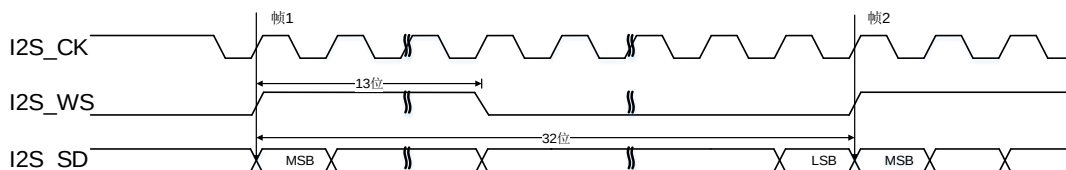
图 22-48. PCM 标准长帧同步模式时序图 (DTLEN=10, CHLEN=1, CKPL=1)
