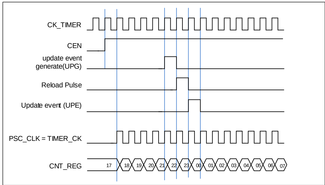
图 17-2. 内部时钟分频为 1 时正常模式下的控制电路
