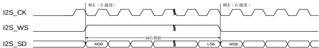
图 22-26. MSB 对齐标准时序图 (DTLEN=00, CHLEN=0, CKPL=1)
