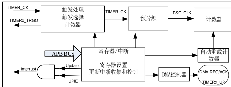
图 17-39. 基本定时器结构框图
