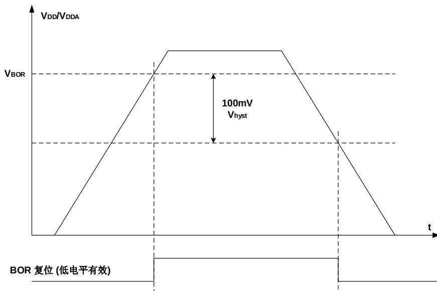
图3-3. BOR波形图
