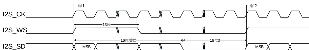
图 22-51. PCM 标准长帧同步模式时序图 (DTLEN=00, CHLEN=1, CKPL=0)
