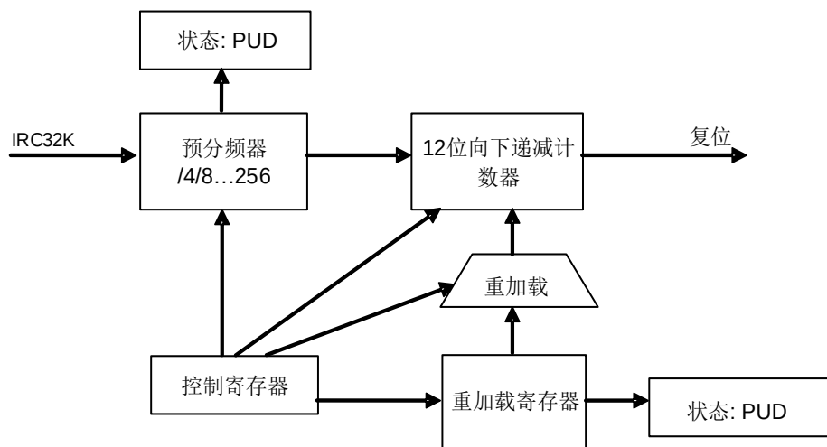
图 15-1. 独立看门狗定时器框图
