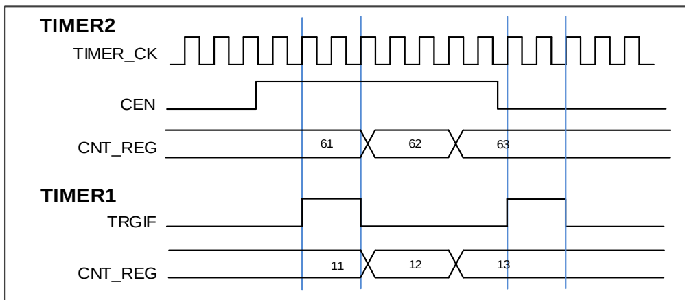
图 17-23. 用定时器 2 的使能信号来控制定时器 1 的暂停模式
