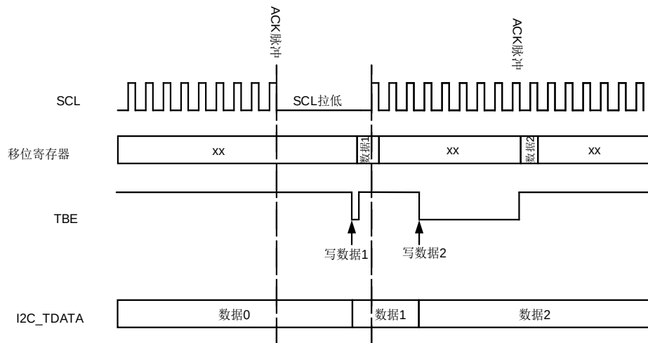
图 21-11. 数据发送
