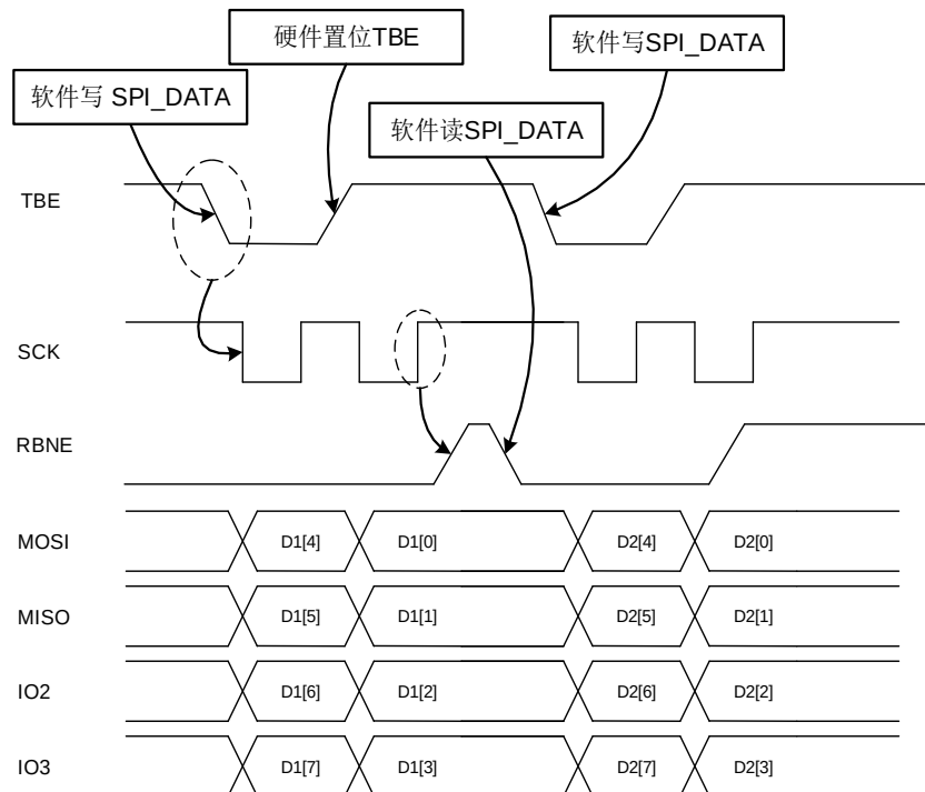
图 22-15. SPI 四线模式四线读操作时序图
