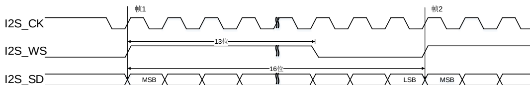
图 22-46. PCM 标准长帧同步模式时序图 (DTLEN=00, CHLEN=0, CKPL=1)
