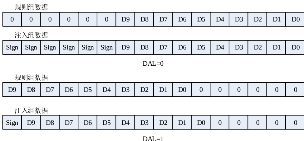
图 13-11. 8 位数据对齐
