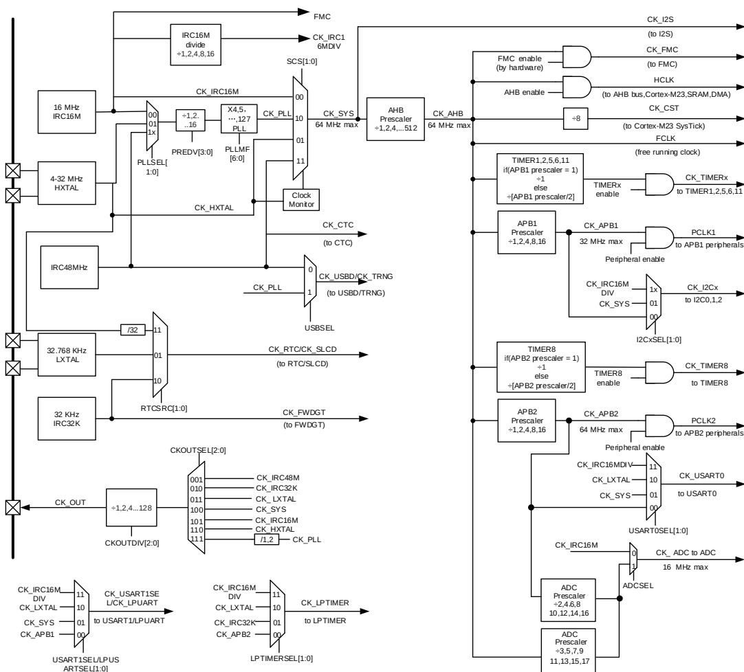
图4-2. 时钟树
