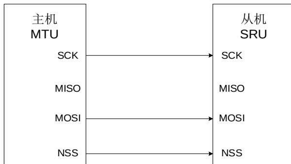
图 22-9. 典型的双向线连接
