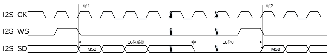
图 22-44. PCM 标准短帧同步模式时序图 (DTLEN=00, CHLEN=1, CKPL=1)
