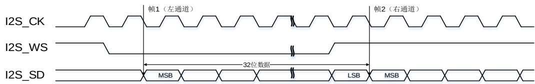
图 22-19. I2S 飞利浦标准时序图 (DTLEN=10, CHLEN=1, CKPL=0)
