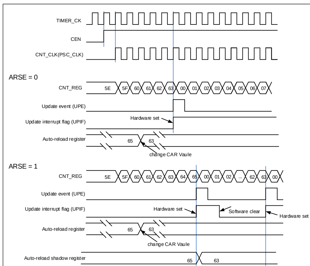
图 17-30. 向上计数时序图, 在运行时改变 TIMERx_CAR 寄存器的值
