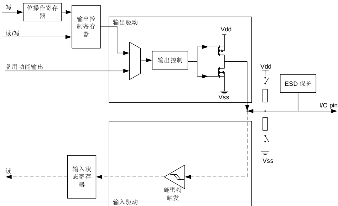
图 7-3. 输出配置
