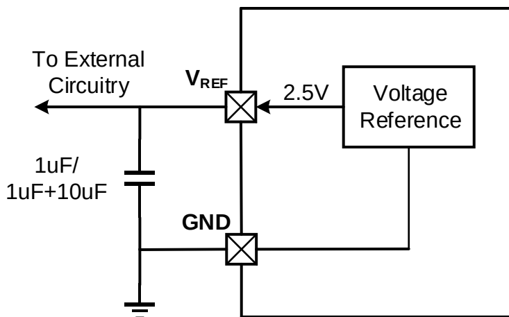
图 24-1. VREF 连接
