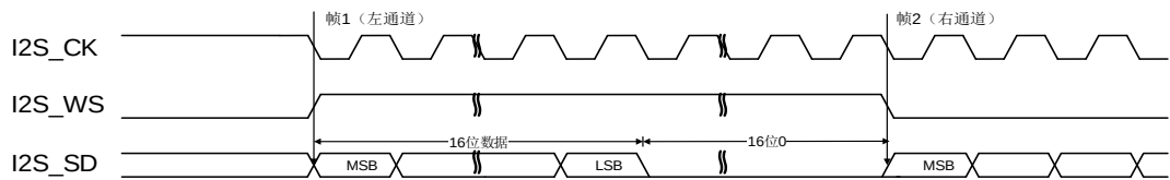
图 22-32. MSB 对齐标准时序图 (DTLEN=00, CHLEN=1, CKPL=1)
