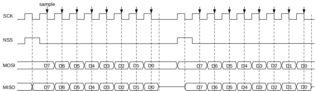
图 22-11. 主机 TI 模式在连续发送时的时序图
