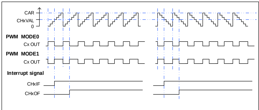
图 17-13. CAPWM 时序图
