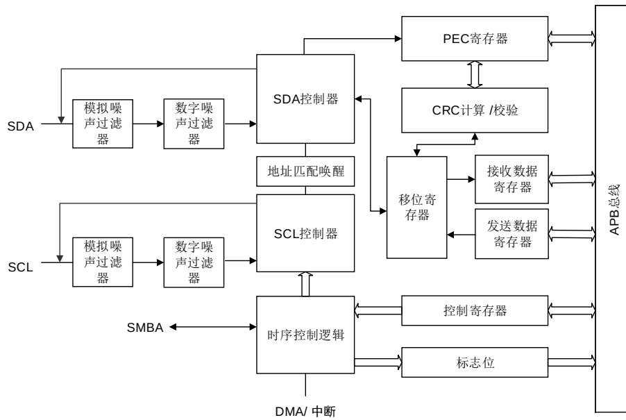
图 21-1. I2C 模块框图
