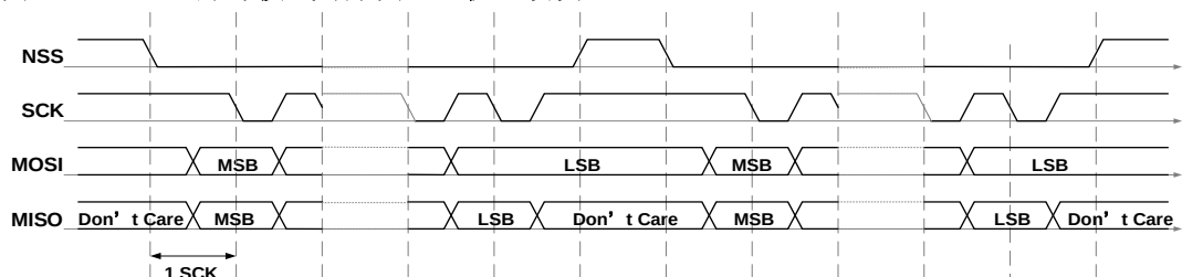
图 22-13. NSS 脉冲模式时序图（主机连续发送）
