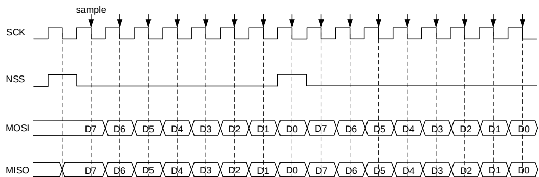
图 22-11. 主机 TI 模式在连续发送时的时序图
