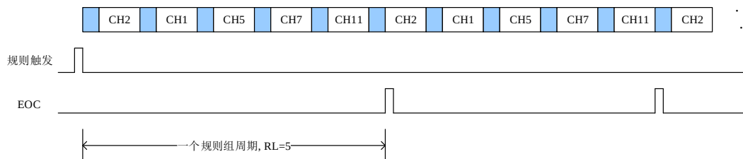
图 13-5. 扫描转换模式，连续转换模式使能
