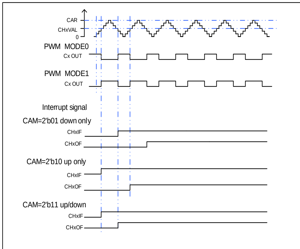
图 17-34. CAPWM 时序图
