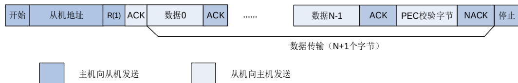
图 21-23. SMBus 主机接收器和从机发送器通信流程
