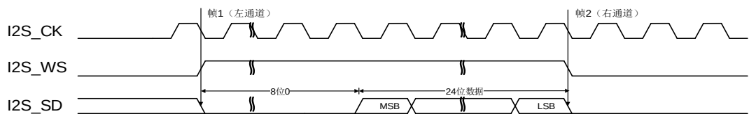
图 22-33. LSB 对齐标准时序图 (DTLEN=01, CHLEN=1, CKPL=0)
