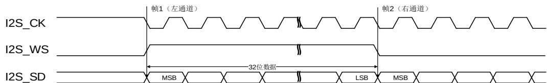
图 22-28. MSB 对齐标准时序图 (DTLEN=10, CHLEN=1, CKPL=1)
