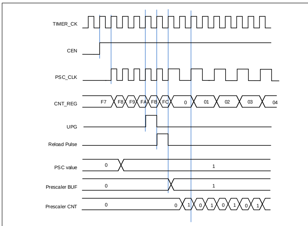
图 17-28. 当预分频器的参数从 1 变到 2 时，计数器的时序图
