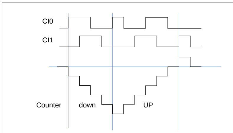
图 17-15. CI0FE0 极性反相的编码器接口模式下的例子
