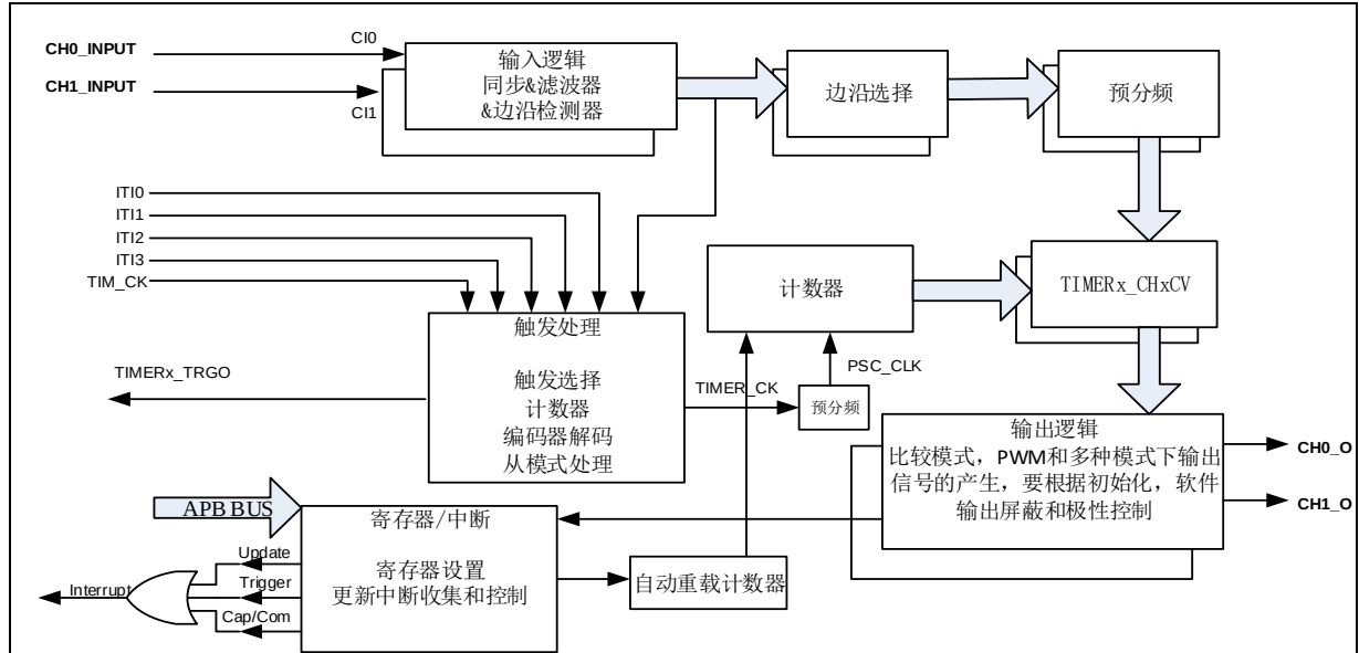
图 17-26. 通用定时器 L1 结构框图
