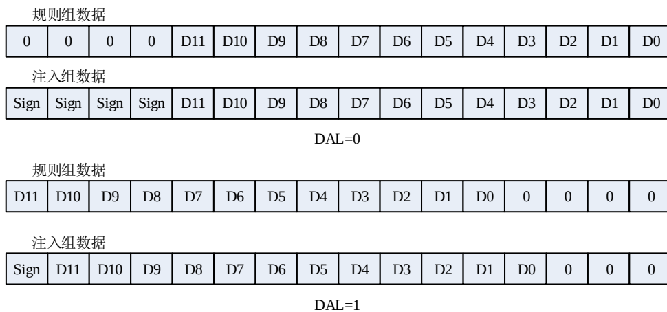
图 13-9. 12 位数据对齐
