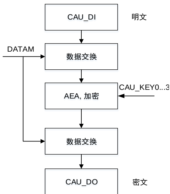
图 23-8. AES ECB 加密
