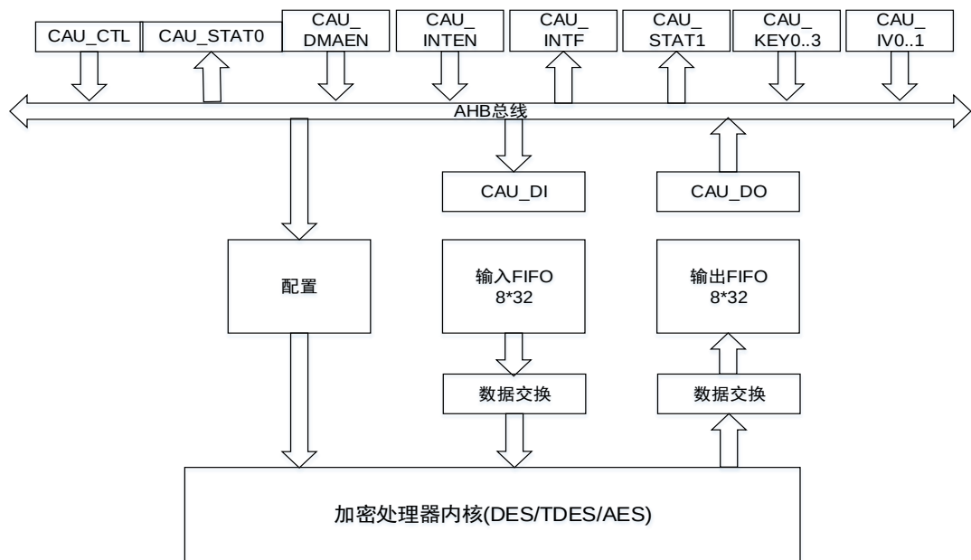
图 23-3. CAU 框图
