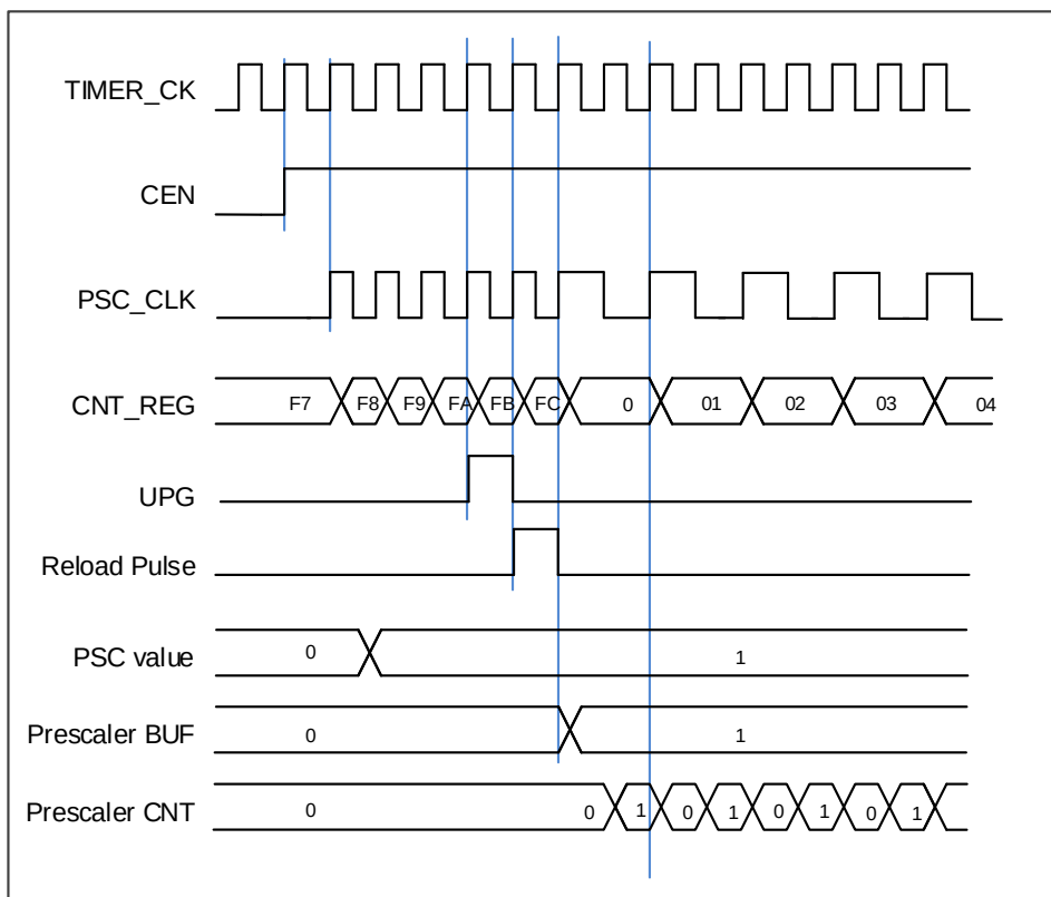
图 17-3. 当预分频器的参数从 1 变到 2 时，计数器的时序图
