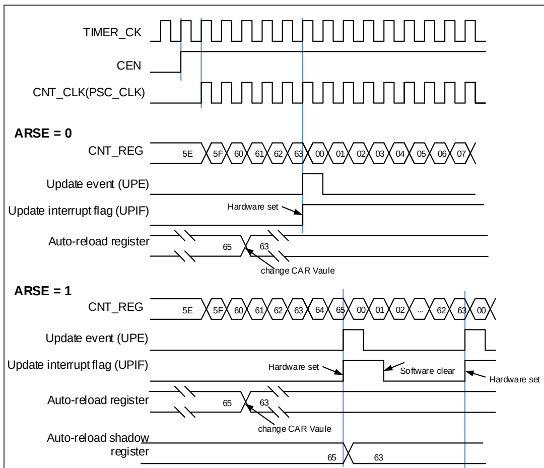
图 17-5. 向上计数时序图，在运行时改变 TIMERx_CAR 寄存器的值
