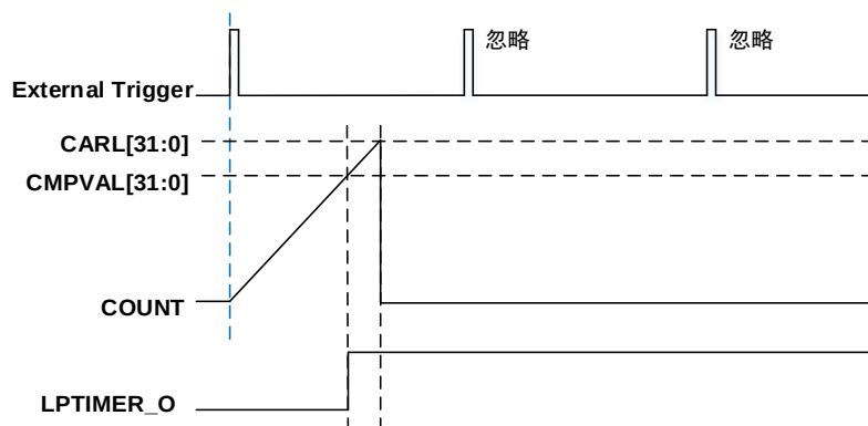
图 18-7. LPTIMER 输出 (OMSEL = 1)
