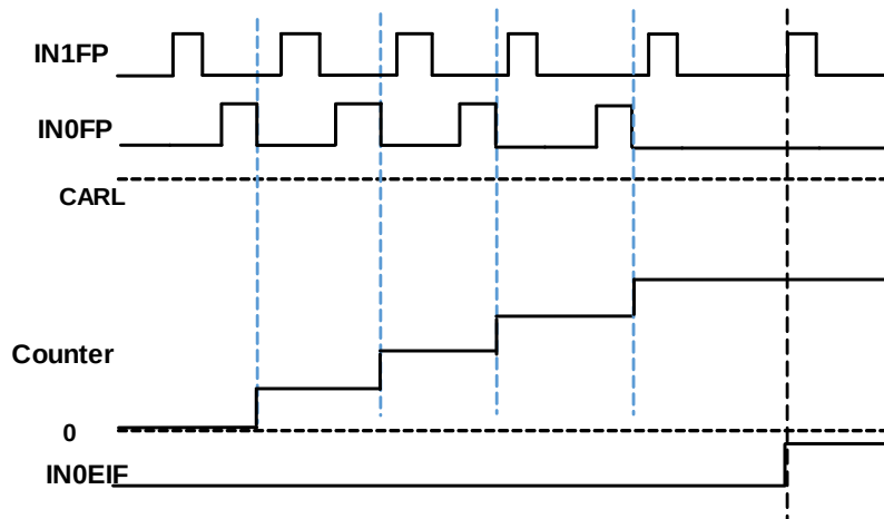
图 18-15. 计数器运行在编码器模式 1（同相，IN0EIF）
