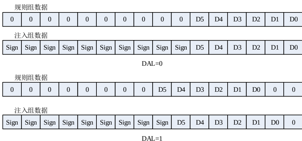
图 13-12. 6 位数据对齐
