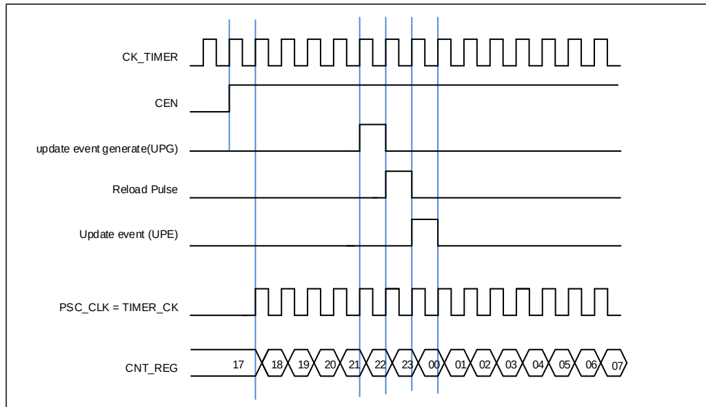
图 17-27. 内部时钟分频为 1 时正常模式下的控制电路
