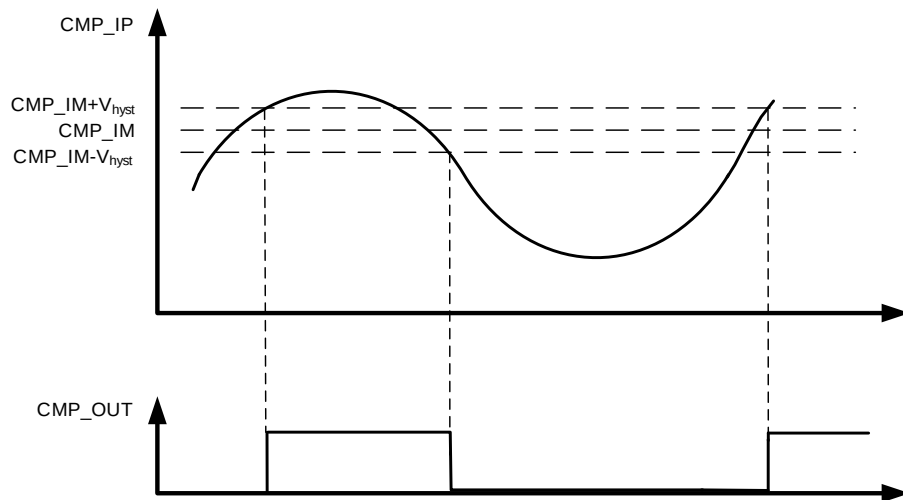
图 26-2. 比较器迟滞
