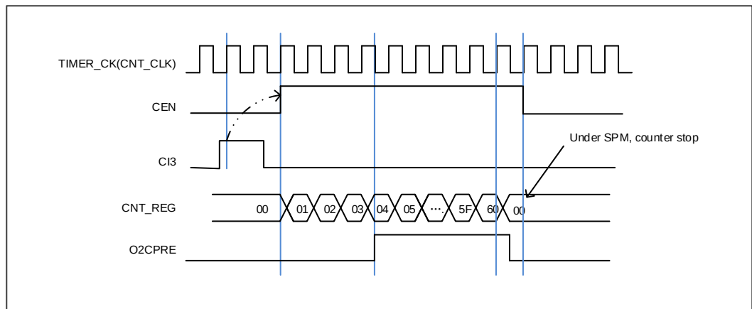
图 17-38. 单脉冲模式， TIMERx_CHxCV = 0x04 TIMERx_CAR=0x60
