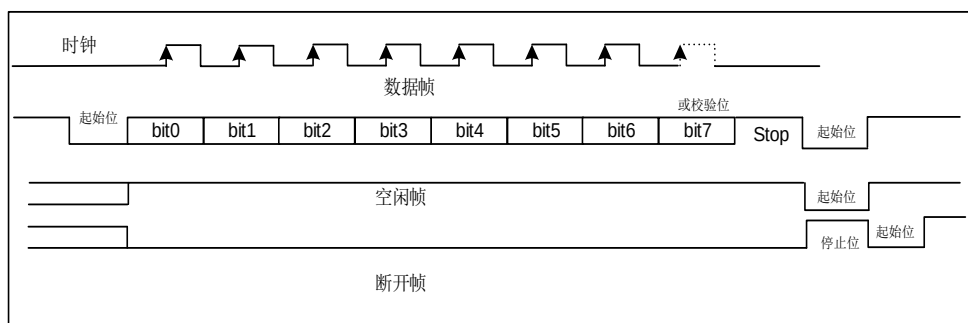
图19-2. USART 字符帧（8数据位和1停止位）
