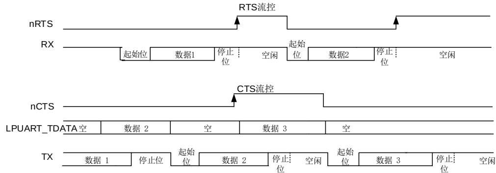
图 20-7. 硬件流控制
