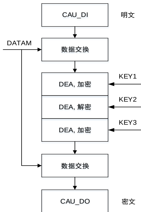
图 23-4. DES/TDES ECB 加密
