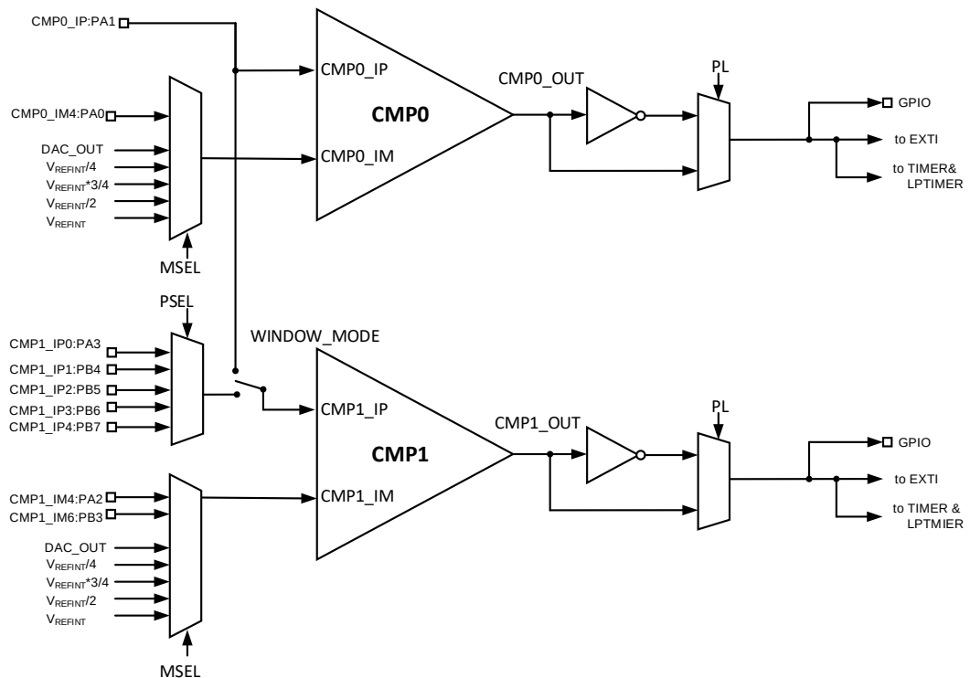
图 26-1 比较器框图
