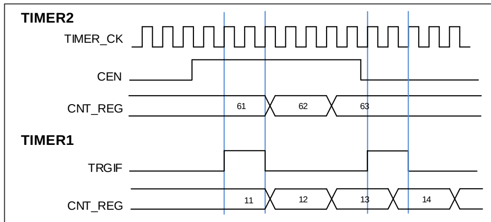
图 17-21. 用定时器 2 的使能信号触发定时器 1
