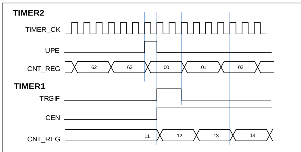
图 17-22. 用定时器 2 的更新事件来触发定时器 1
