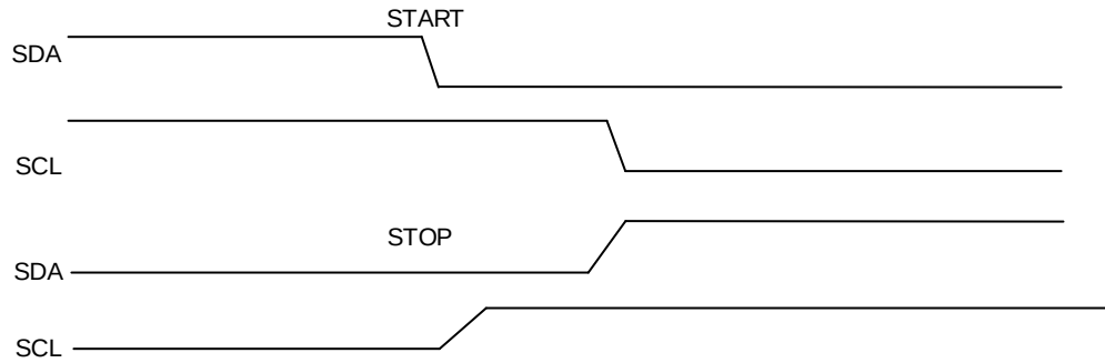
图 21-3. 开始和停止状态
