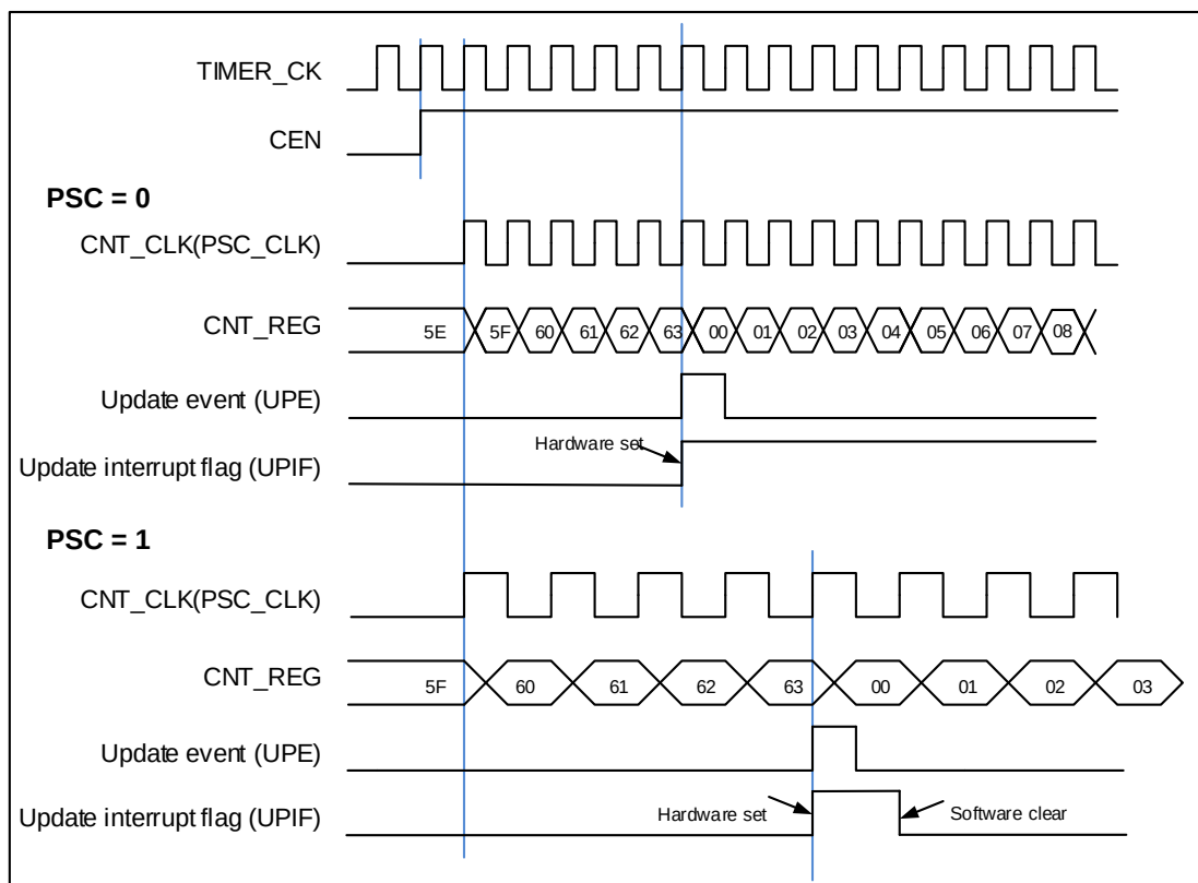
图 17-4. 向上计数时序图, PSC=0/1
