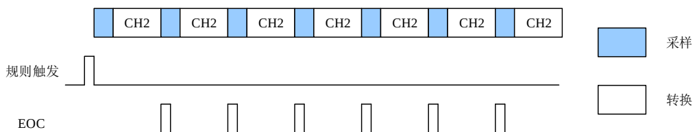
图 13-3. 连续转换模式
