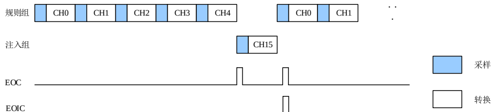
图 13-7. 自动注入，CTN=1
