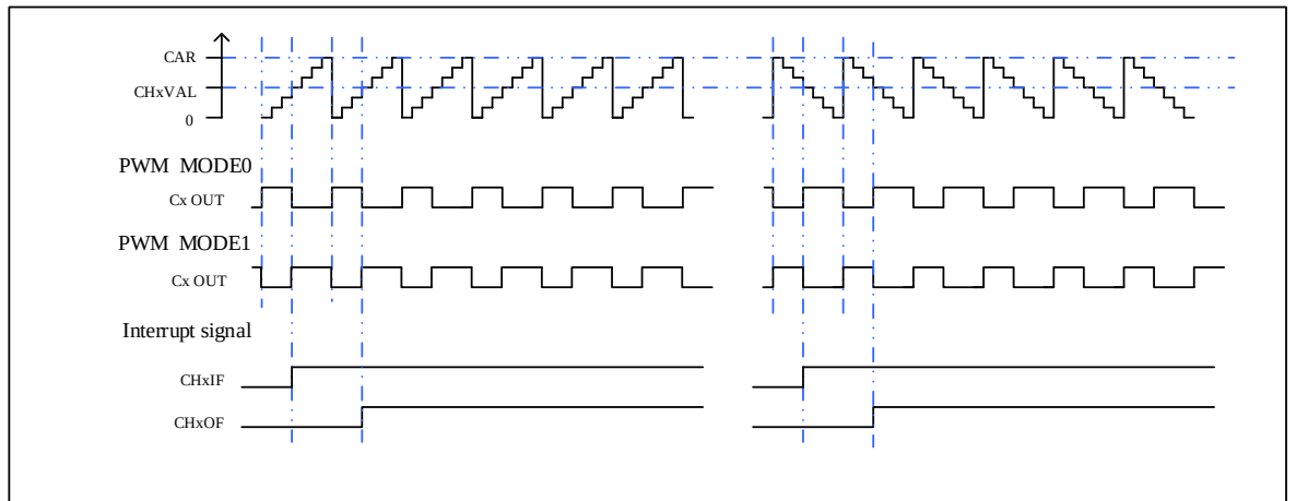
图 17-33. EAPWM 时序图
