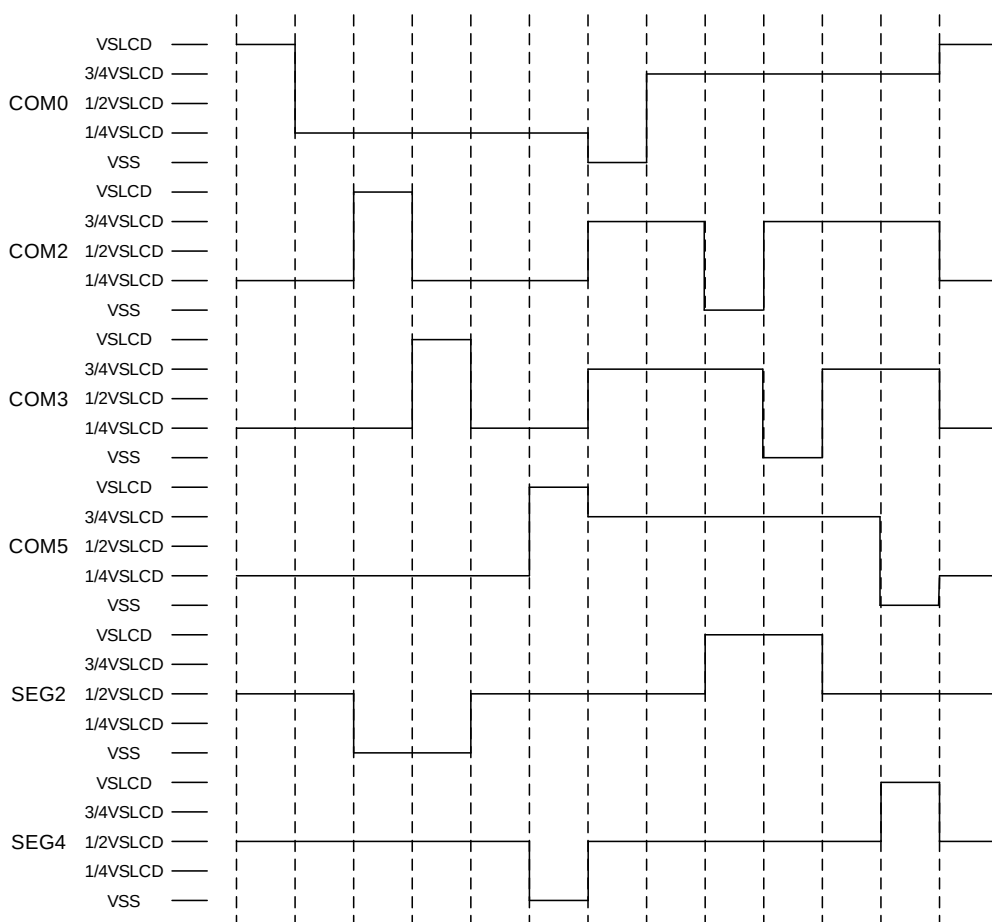
图 25-3. 1/4 偏置 1/6 占空比
