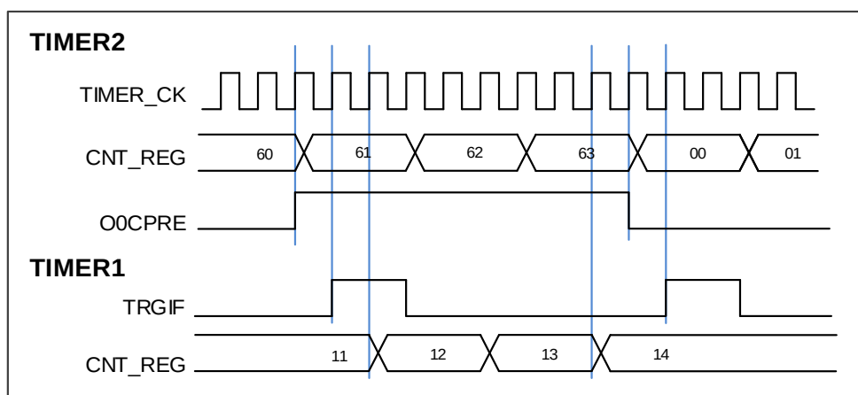
图 17-24. 用定时器 2 的 O0CPRE 信号控制定时器 1 的暂停模式
