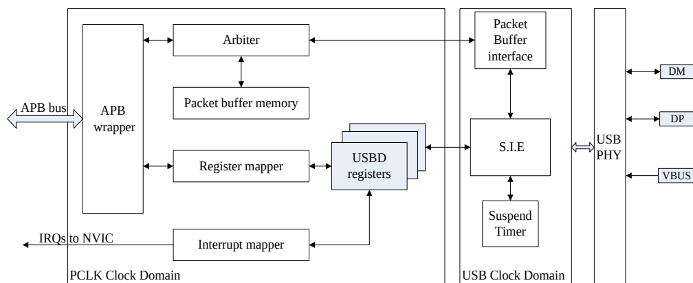
图 27-1. USBD 模块图
