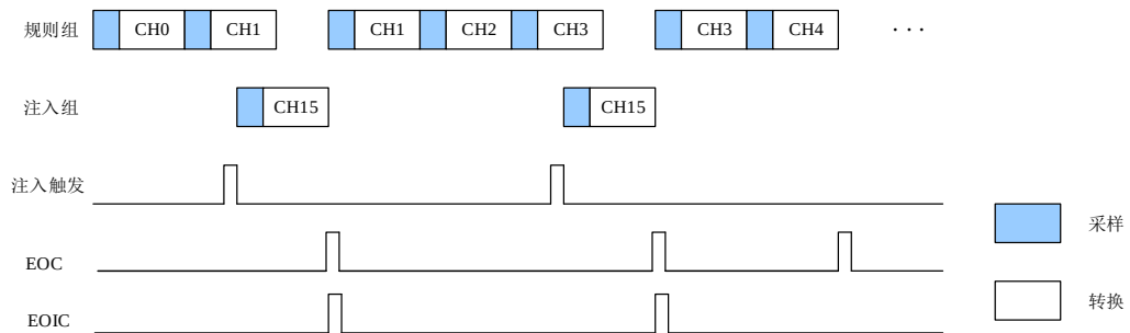
图 13-8. 触发注入
