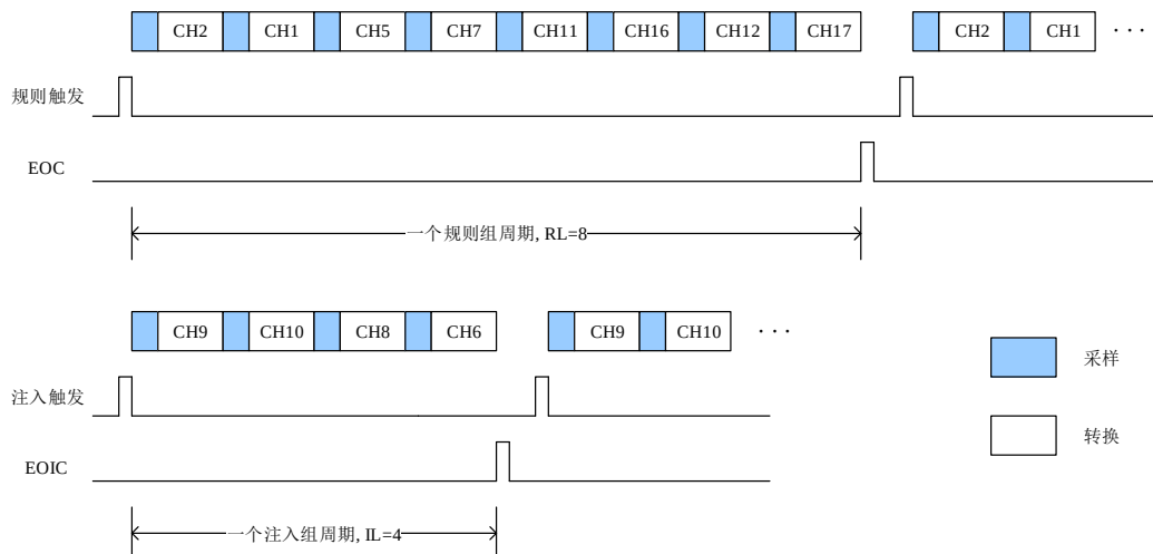
图 13-4. 扫描转换模式，且连续转换模式失能
