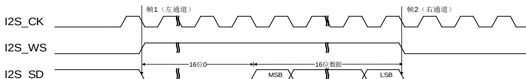
图 22-35. LSB 对齐标准时序图 (DTLEN=00, CHLEN=1, CKPL=0)
