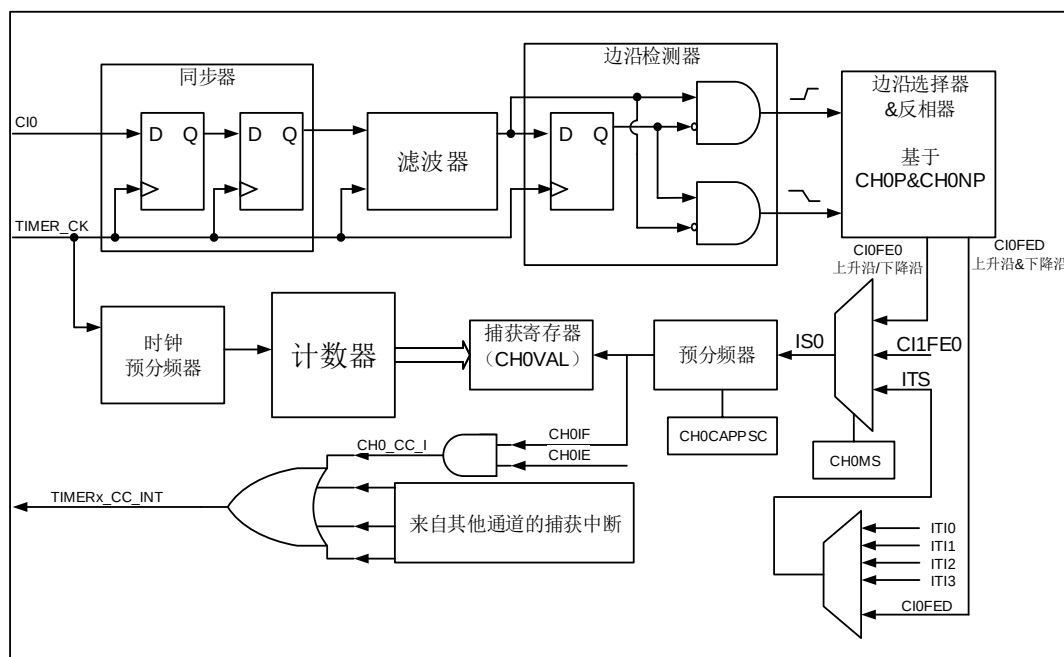
图 17-9. 输入捕获逻辑
