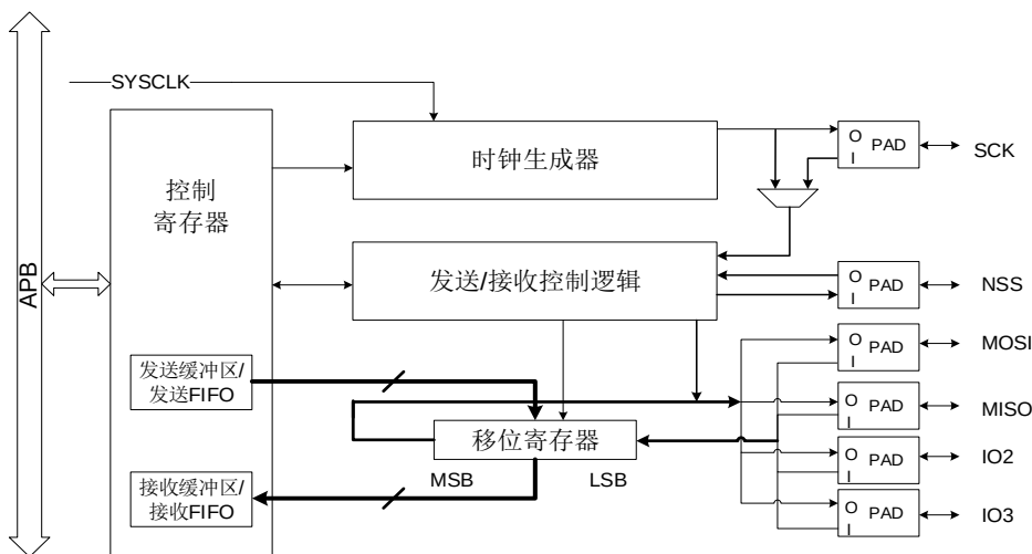
图 22-1. SPI 结构框图
