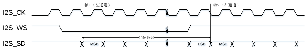
图 22-17. I2S 飞利浦标准时序图（DTLEN=00, CHLEN=0, CKPL=0）
