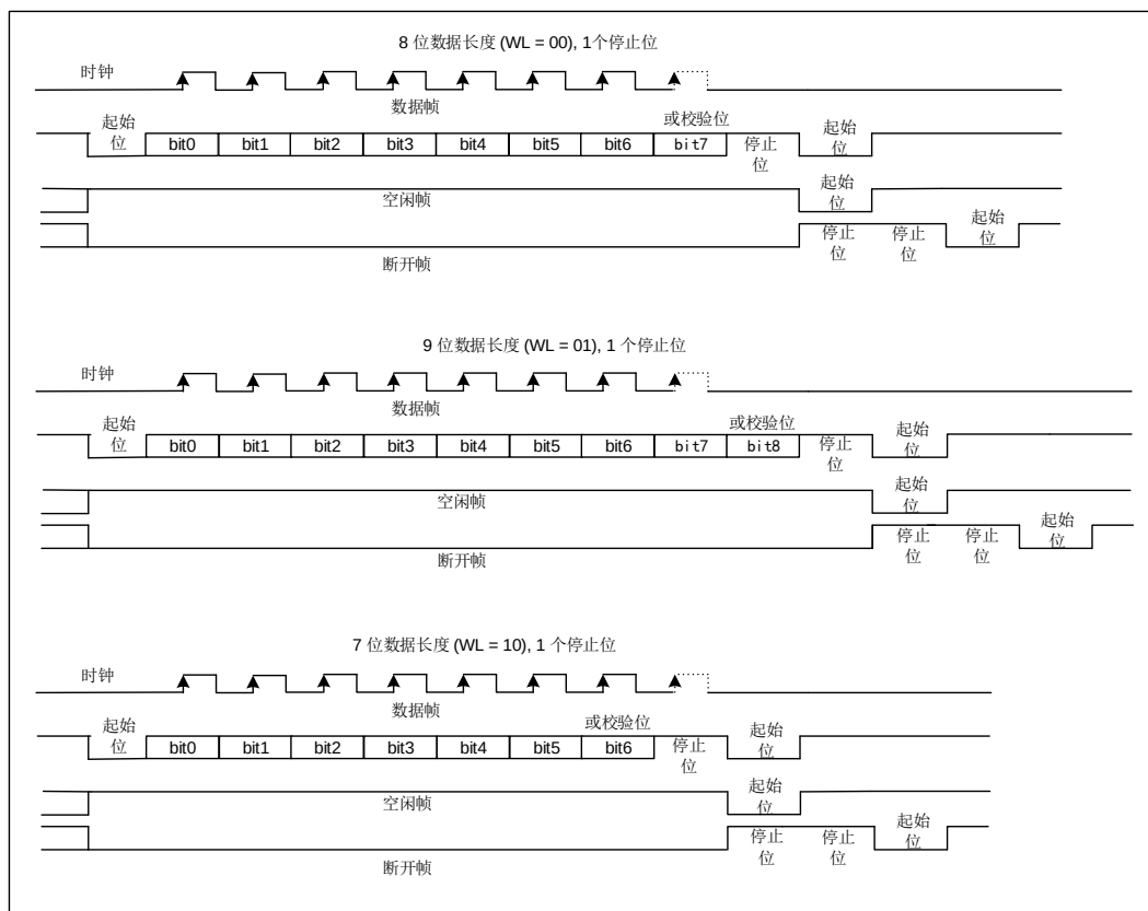
图20-2. LPUART字符帧
