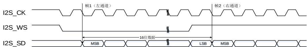
图 22-18. I2S 飞利浦标准时序图（DTLEN=00, CHLEN=0, CKPL=1）
