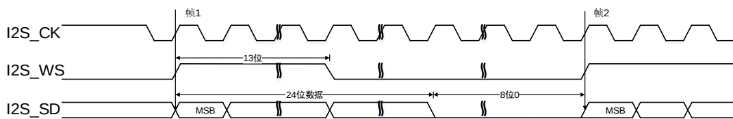
图 22-50. PCM 标准长帧同步模式时序图 (DTLEN=01, CHLEN=1, CKPL=1)
