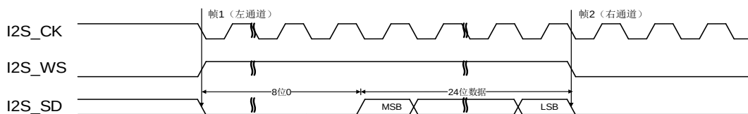
图 22-34. LSB 对齐标准时序图 (DTLEN=01, CHLEN=1, CKPL=1)
