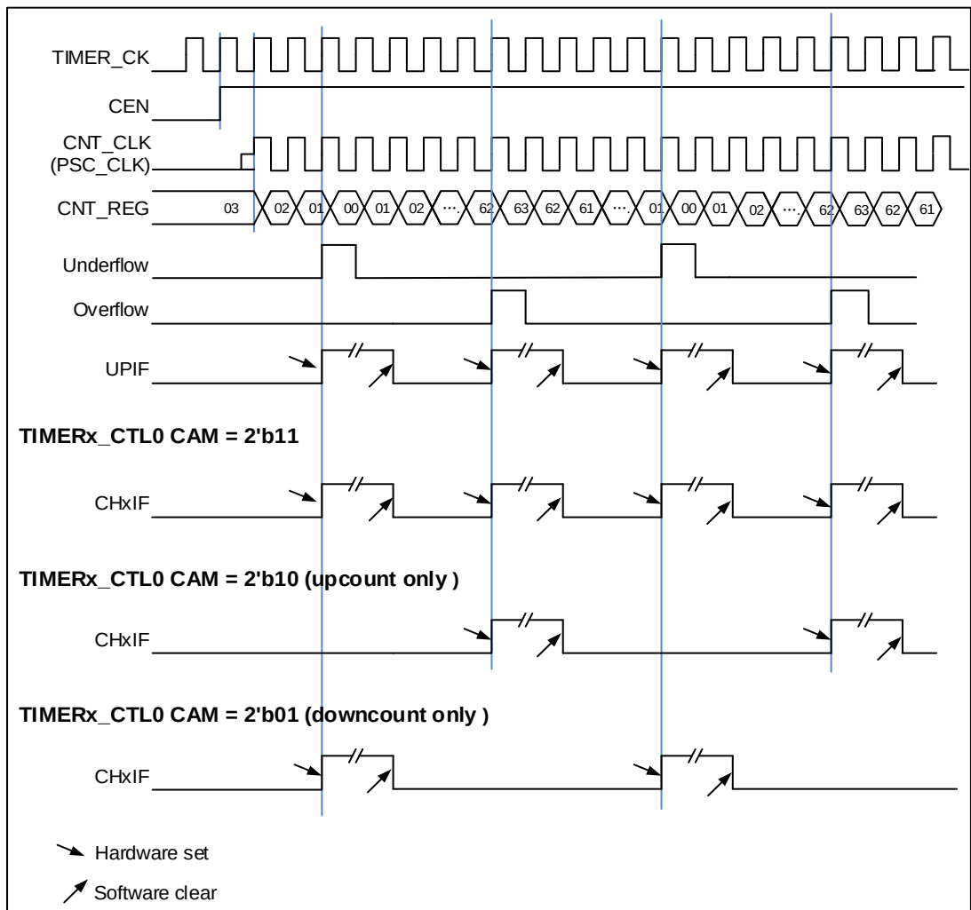
图 17-8. 中央计数模式计数器时序图
