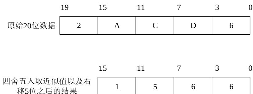
图 13-14. 右移 5 位和取整的数例
