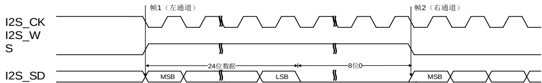
图 22-30. MSB 对齐标准时序图 (DTLEN=01, CHLEN=1, CKPL=1)
