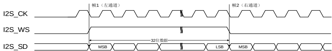
图 22-27. MSB 对齐标准时序图 (DTLEN=10, CHLEN=1, CKPL=0)
