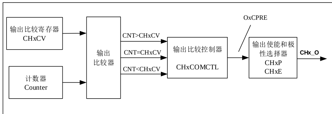
图 17-10. 输出比较逻辑 ( x=0, 1, 2, 3 )
