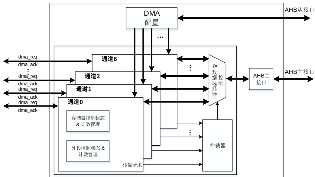
图 10-1. DMA 结构框图
