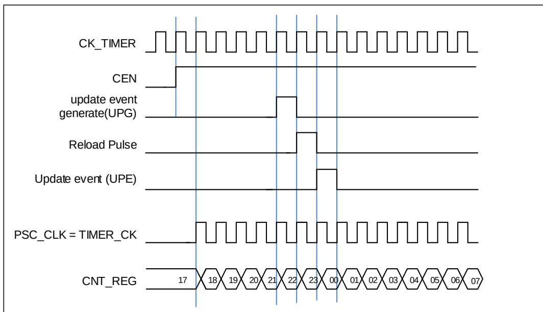
图 17-40. 内部时钟分频为 1 时正常模式下的控制电路
