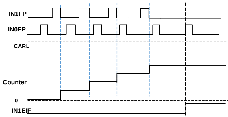
图 18-14. 计数器运行在编码器模式 1（同相，IN1EIF）
