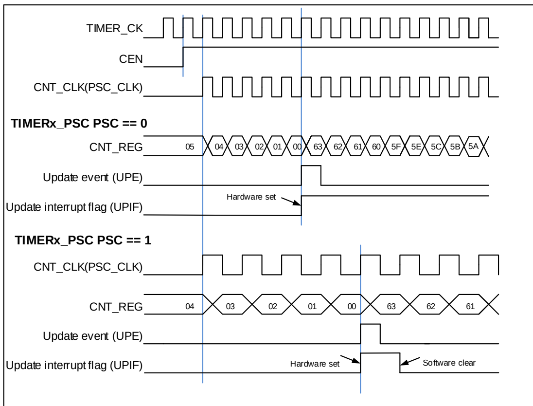
图 17-6. 向下计数时序图, PSC=0/1
