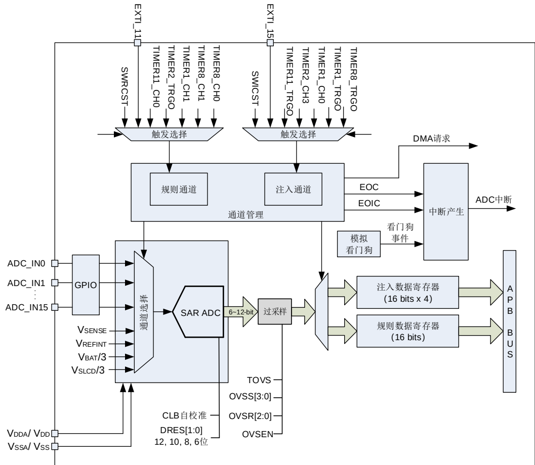
图 13-1. ADC 模块框图
