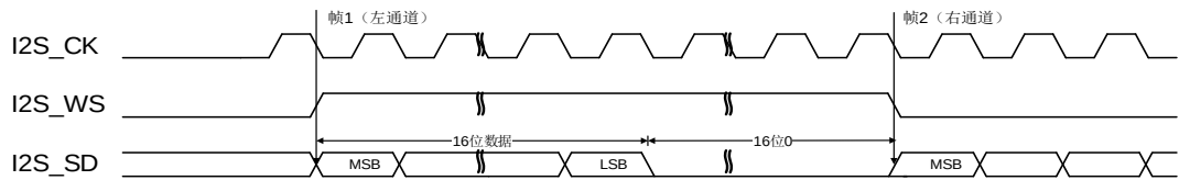
图 22-31. MSB 对齐标准时序图 (DTLEN=00, CHLEN=1, CKPL=0)
