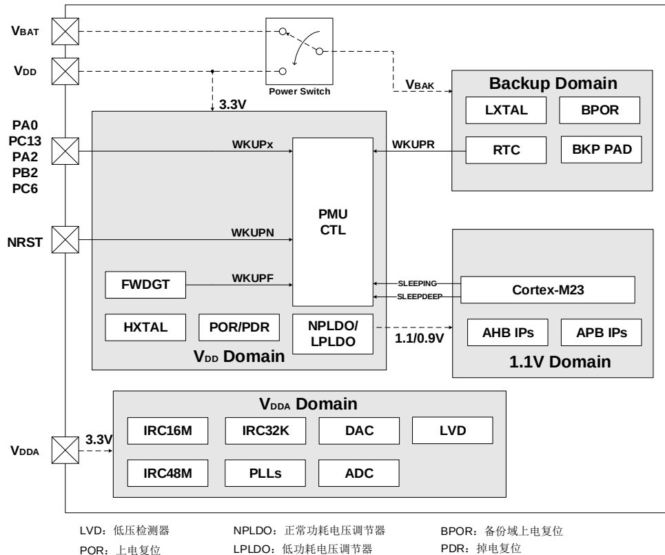
图3-1. 电源域概览
