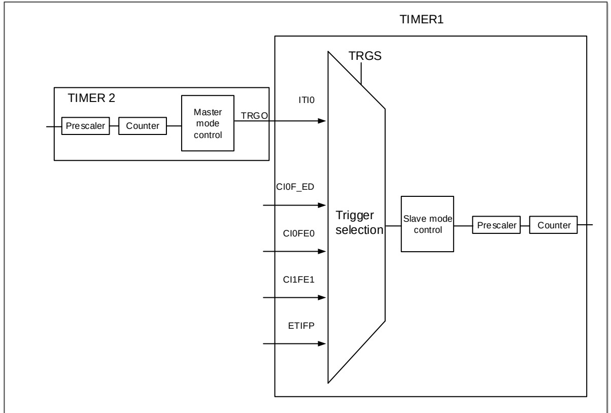
图 17-20. 定时器 1 主/从模式的例子
