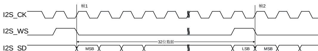
图 22-40. PCM 标准短帧同步模式时序图 (DTLEN=10, CHLEN=1, CKPL=1)
