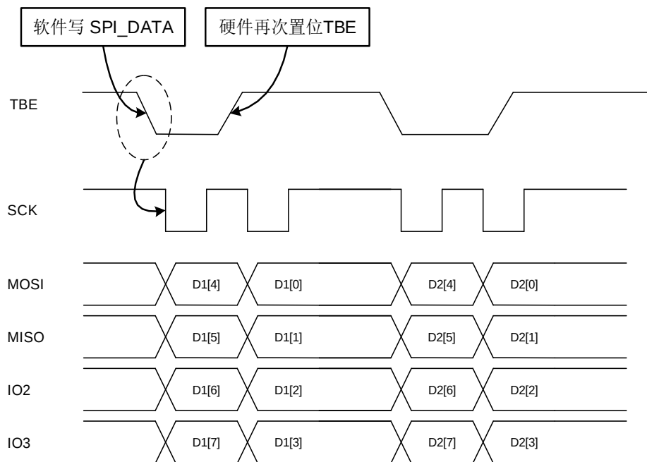
图 22-14. SPI 四线模式四线写操作时序图
