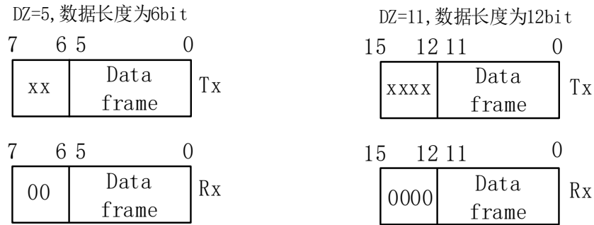
图 22-3. SPI0 数据帧右对齐示意图
