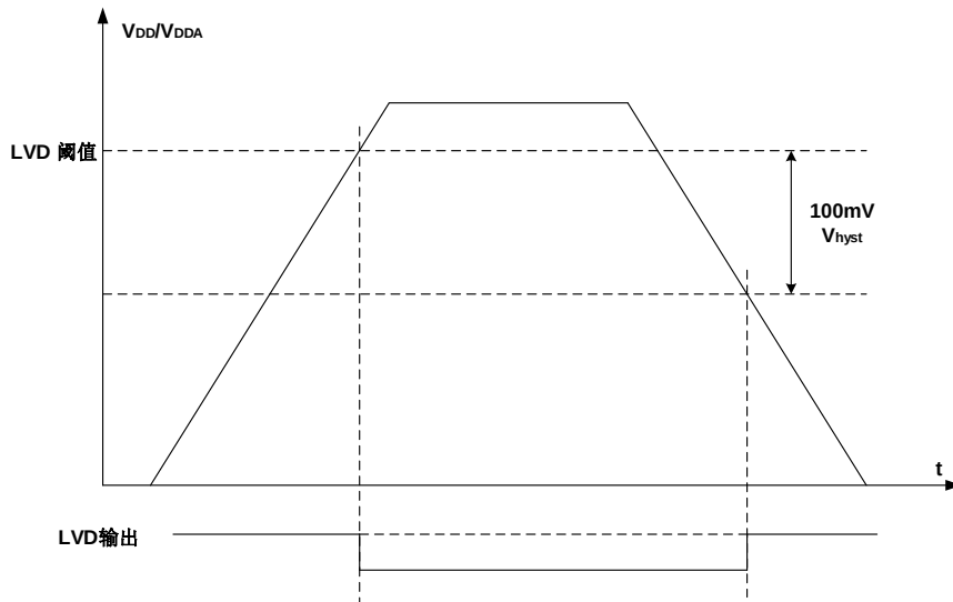
图 3-4. LVD 阈值波形图
