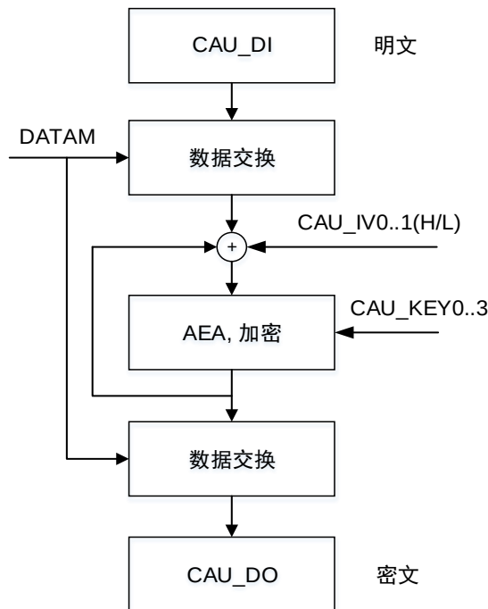
图 23-10. AES CBC 加密
