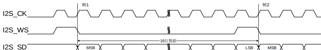
图 22-37. PCM 标准短帧同步模式时序图 (DTLEN=00, CHLEN=0, CKPL=0)
