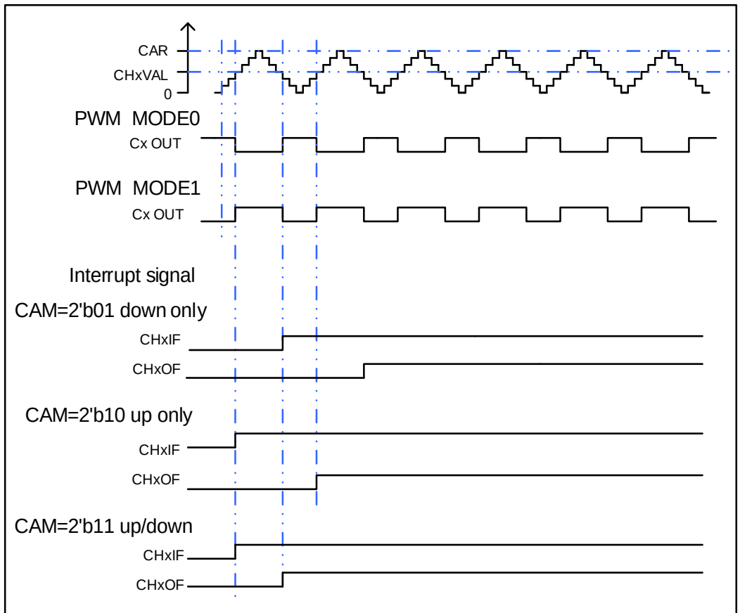
图 17-13. CAPWM 时序图
