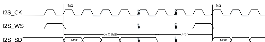
图 22-41. PCM 标准短帧同步模式时序图 (DTLEN=01, CHLEN=1, CKPL=0)
