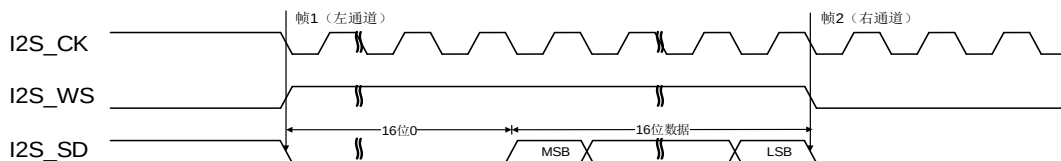
图 22-36. LSB 对齐标准时序图 (DTLEN=00, CHLEN=1, CKPL=1)
