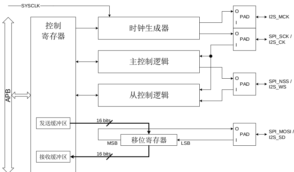
图 22-16. I2S 结构框图
