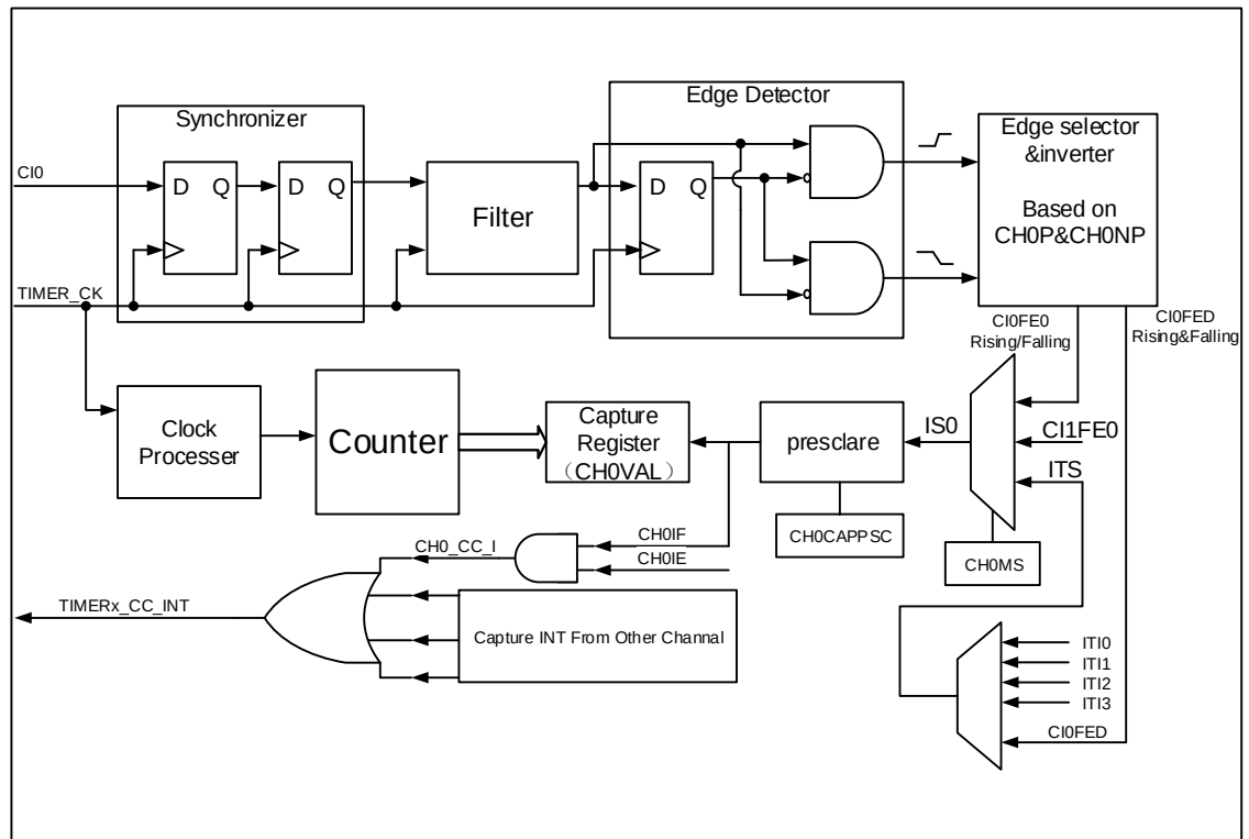
图 17-31. 输入捕获逻辑
