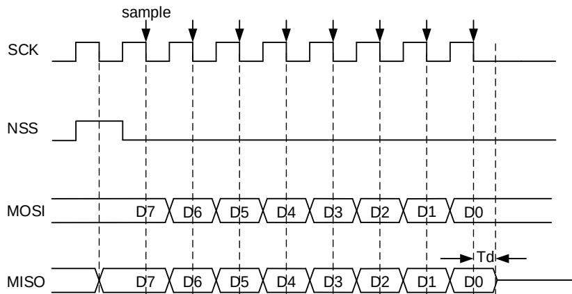
图 22-12. 从机 TI 模式时序图
