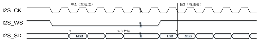
图 22-20. I2S 飞利浦标准时序图 (DTLEN=10, CHLEN=1, CKPL=1)
