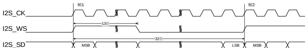
图 22-47. PCM 标准长帧同步模式时序图 (DTLEN=10, CHLEN=1, CKPL=0)
