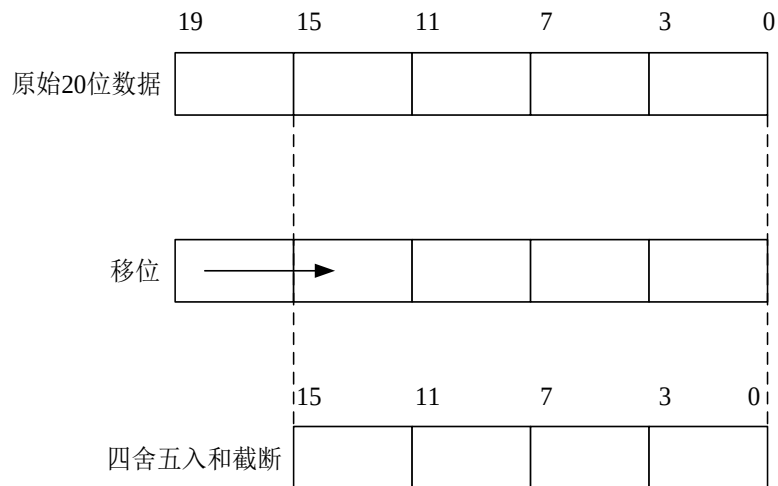
图 13-13. 20 位到 16 位的结果截断
