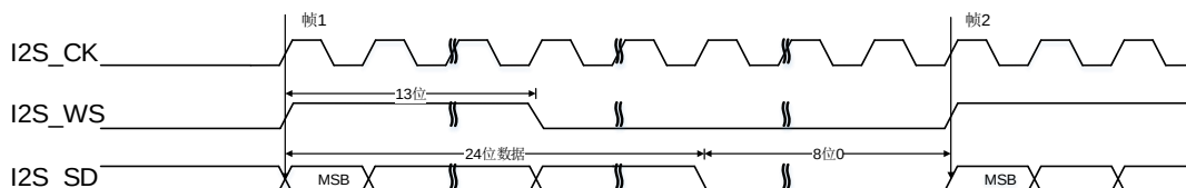
图 22-49. PCM 标准长帧同步模式时序图 (DTLEN=01, CHLEN=1, CKPL=0)
