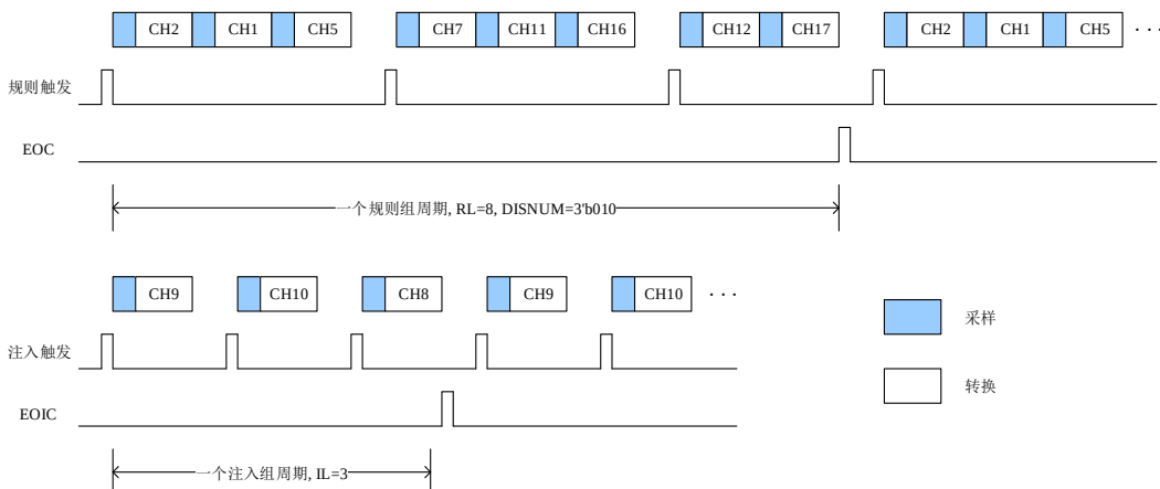
图 13-6. 间断转换模式
