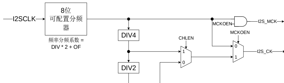
图 22-53. I2S 时钟生成结构框图
