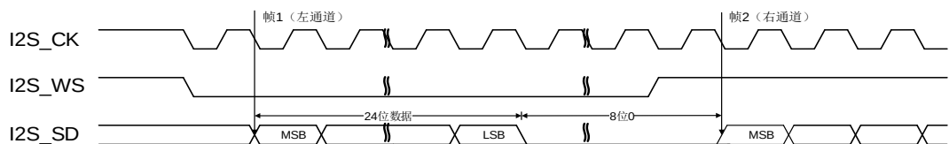
图 22-22. I2S 飞利浦标准时序图 (DTLEN=01, CHLEN=1, CKPL=1)
