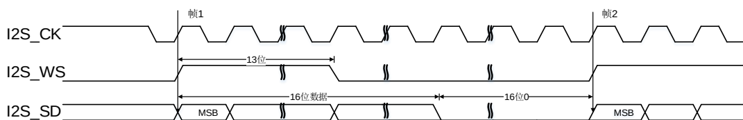
图 22-52. PCM 标准长帧同步模式时序图 (DTLEN=00, CHLEN=1, CKPL=1)
