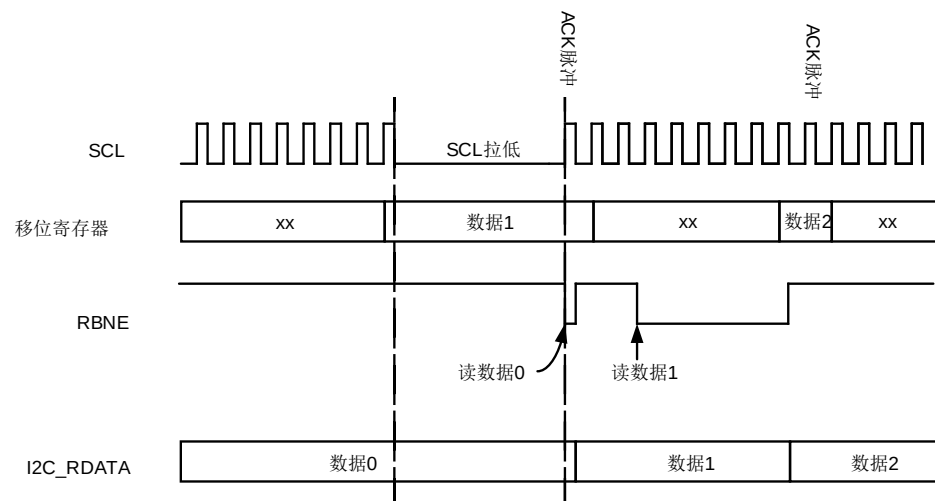
图 21-12. 数据接收
