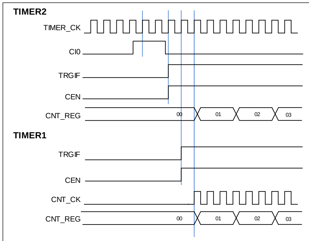
图 17-25. 用定时器 2 的 CI0 信号来触发定时器 1 和定时器 2
