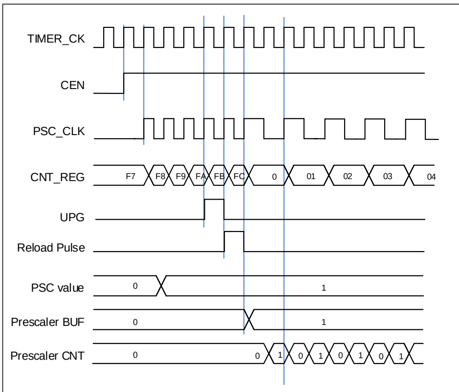
图 17-41. 当预分频器的参数从 1 变到 2 时，计数器的时序图
