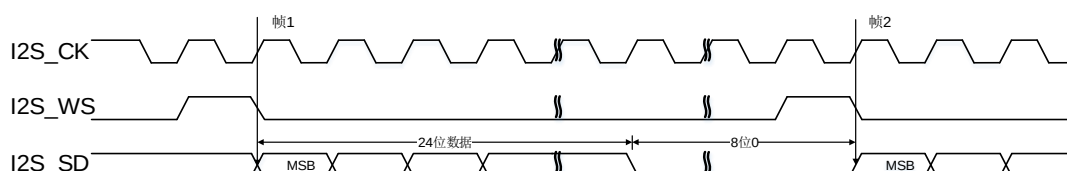
图 22-42. PCM 标准短帧同步模式时序图 (DTLEN=01, CHLEN=1, CKPL=1)
