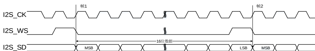
图 22-38. PCM 标准短帧同步模式时序图 (DTLEN=00, CHLEN=0, CKPL=1)
