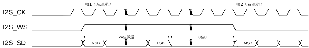
图 22-29. MSB 对齐标准时序图 (DTLEN=01, CHLEN=1, CKPL=0)
