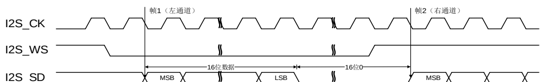
图 22-23. I2S 飞利浦标准时序图 (DTLEN=00, CHLEN=1, CKPL=0)
