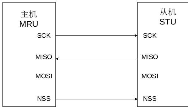
图 22-8. 典型的单工模式连接（主机：只发送，从机：接收）
