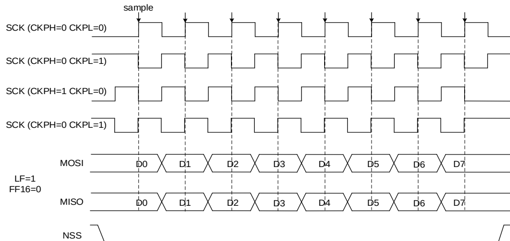
图 22-4. SPI1 常规模式下的时序图
