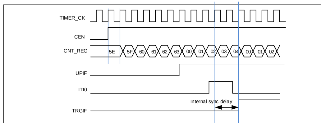
图 17-35. 复位模式下的控制电路
