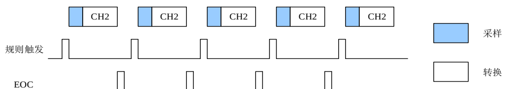
图 13-2. 单次转换模式
