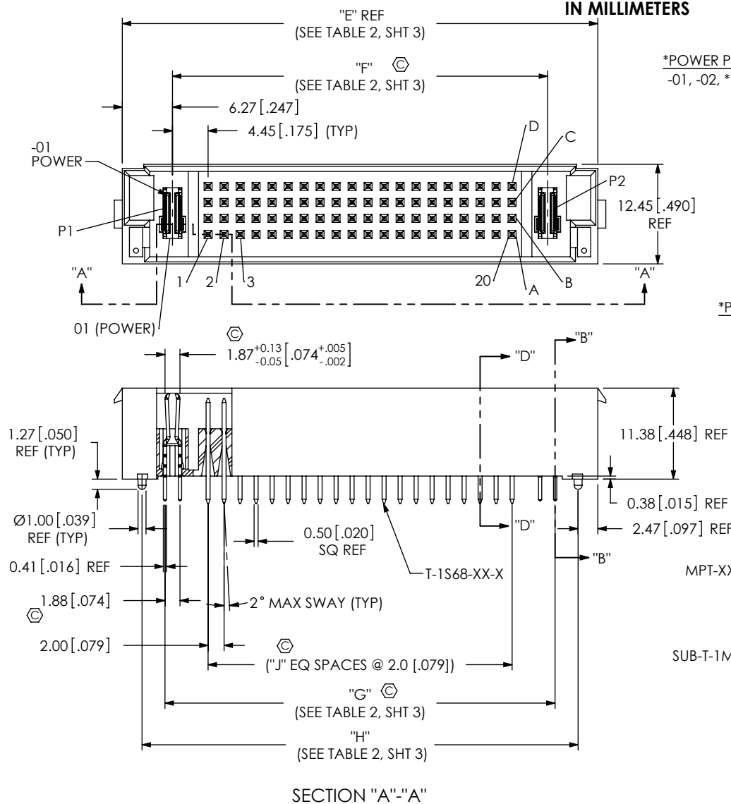
FIG 1 MPTC-01-80-01-6.30-01-X-V SHOWN
