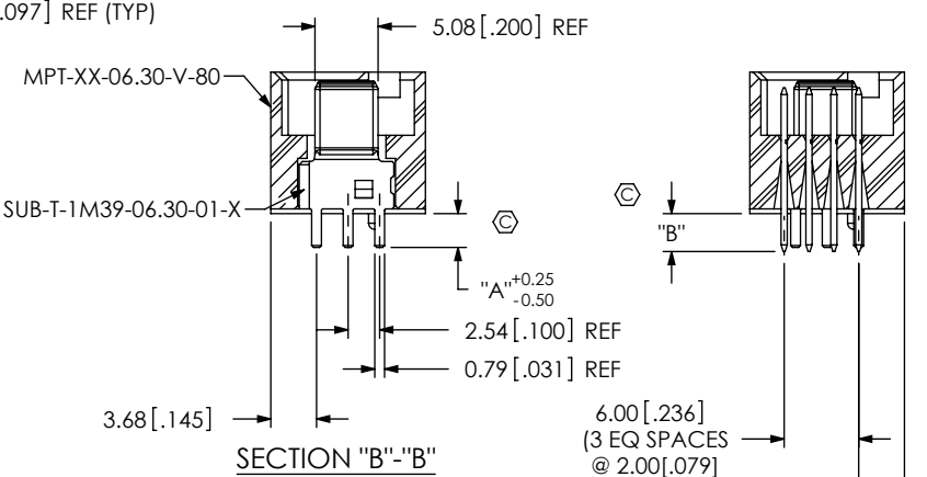
FIG 1 MPTC-01-80-01-6.30-01-X-V SHOWN
