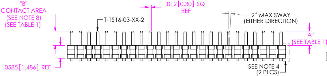
FIG 1 FTMH-125-03-X-DV SHOWN
