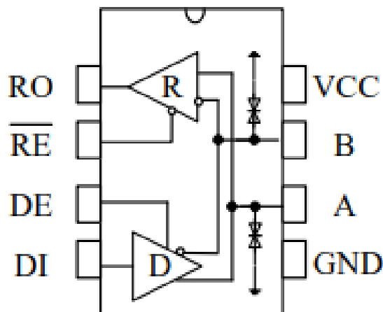
图 1 SN65HVD485EDR 引脚分布图
