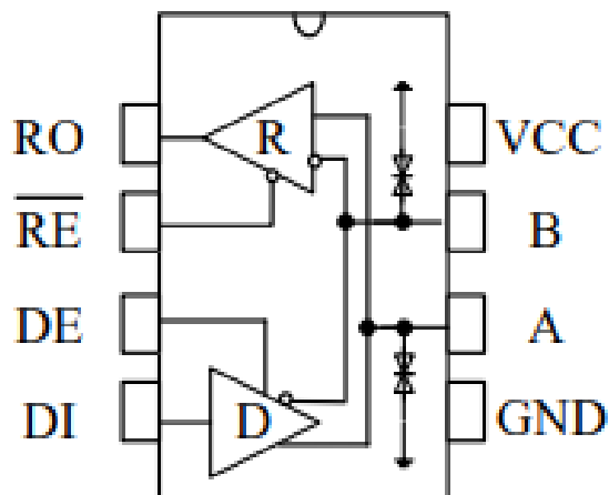
图 1 SN65HVD82DR 引脚分布图
