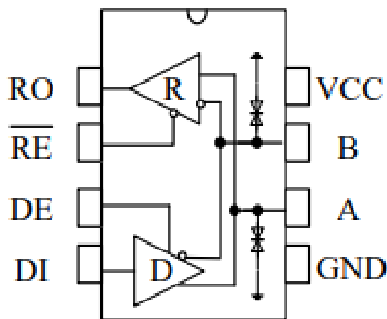
图 1 MAX3485ESA+T 引脚分布图
